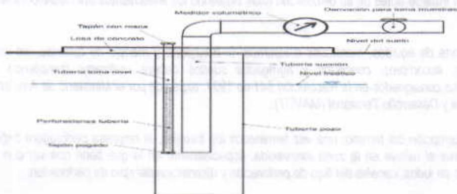
Figura 2. Instalación dispositivos de control al pozo
