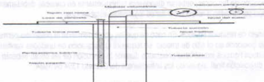
Figura 2. Instalación dispositivos de control al pozo
