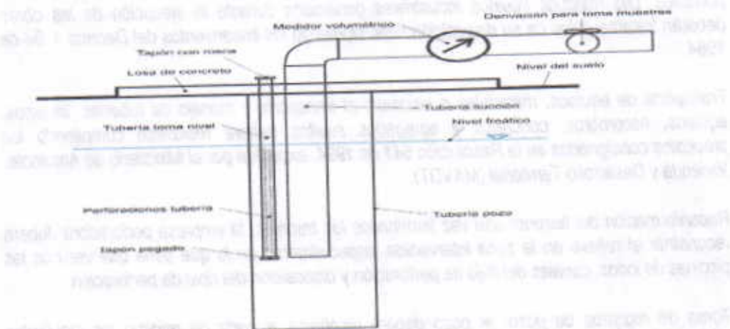
Figura 2. Instalación dispositivos de control al pozo
