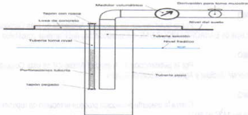
Figura 2. Instalación dispositivos de control pozos
