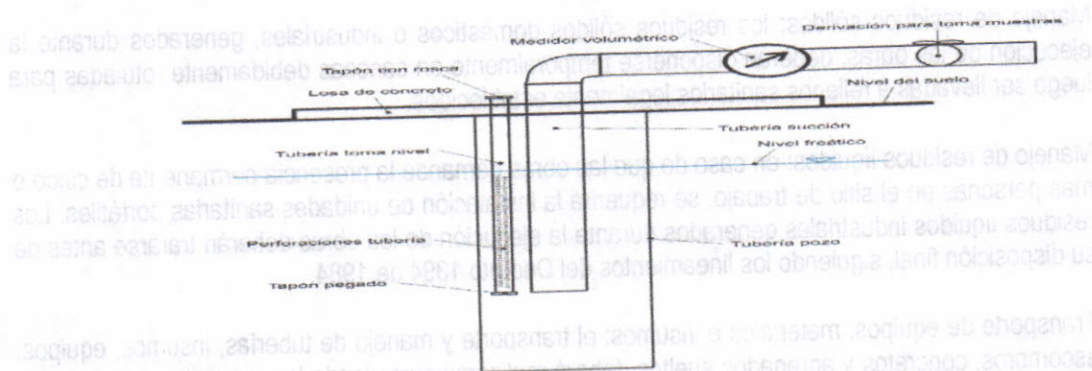
Figura 2. Instalación dispositivos de control al pozo
