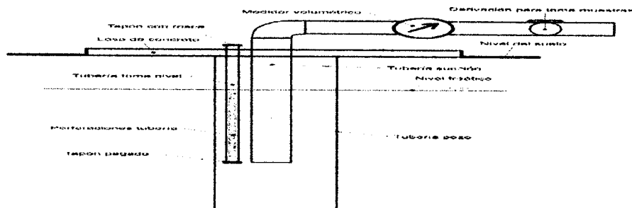
Figura 2 Instalación dispositivos de control al pozo
