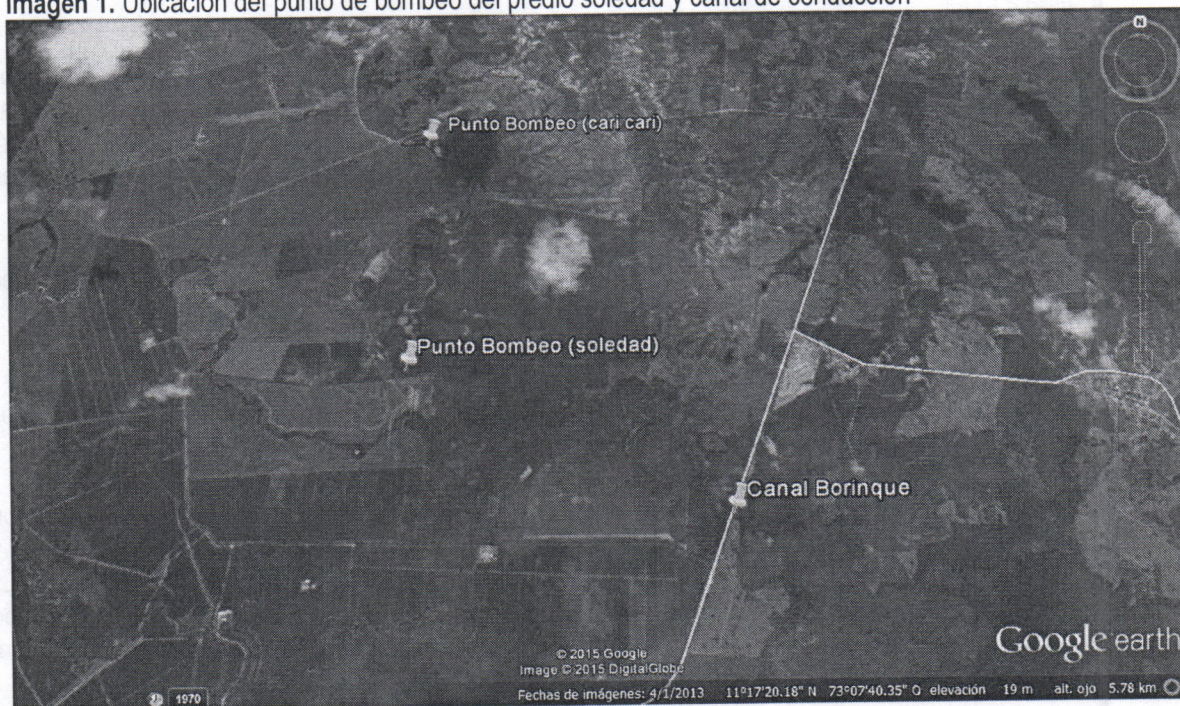
Imagen 1. Ubicación del punto de bombeo del predio soledad y canal de conducción
