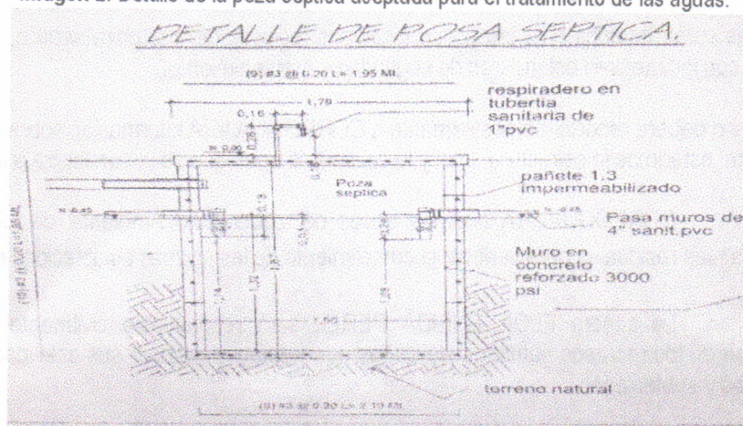
Imagen 2. Detalle de la poza séptica aceptada para el tratamiento de las aguas.
