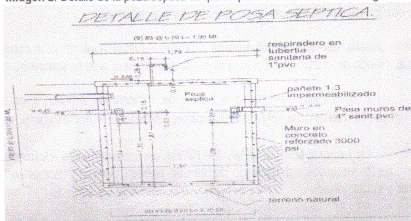
Imagen 2. Detalle de la poza séptica aceptada para el tratamiento de las aguas.
