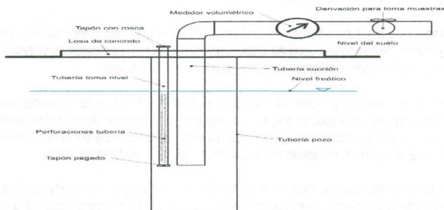
Figura 2. Instalación dispositivos de control al pozo
