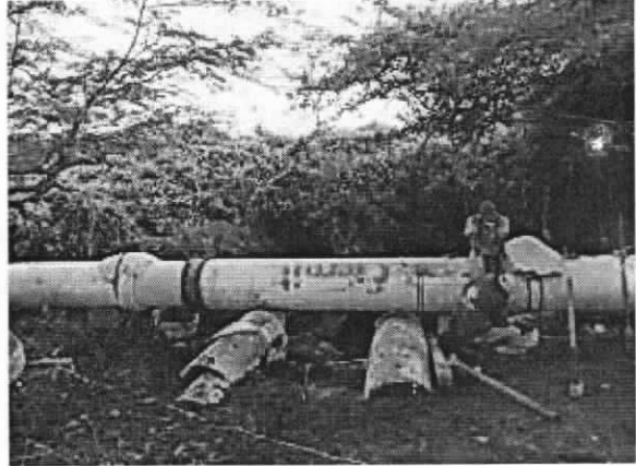
Fotografías No 9, 10, 11 y 12. Reparaciones en la tubería de conducción del agua residual hasta el sistema de tratamiento aguas residuales del municipio de maicao (Laguna de oxidación). Sistema de tratamiento de aguas residuales de Maicao. Seguimiento ambiental realizado el 12/10/2016
