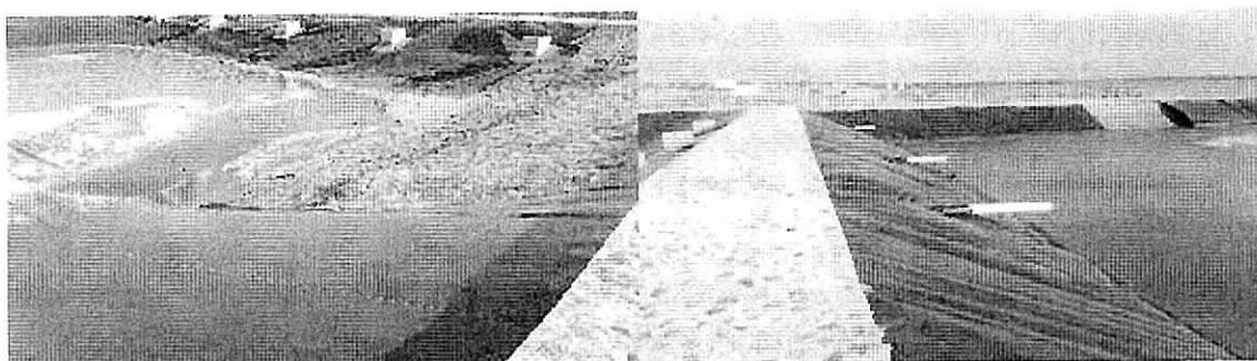
Fotografías No 3 – 6. Membrana impermeable levantada o inexistente en algunos tramos del sistema de tratamiento de aguas residuales del corregimiento de El Pájaro.
