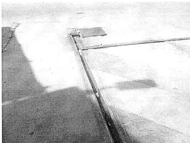
Foto No 2: Canales perimetrales y cajilla colectora. EDS EL PROGRESO PEÑA. Maicao, 15 de diciembre de 2017.
