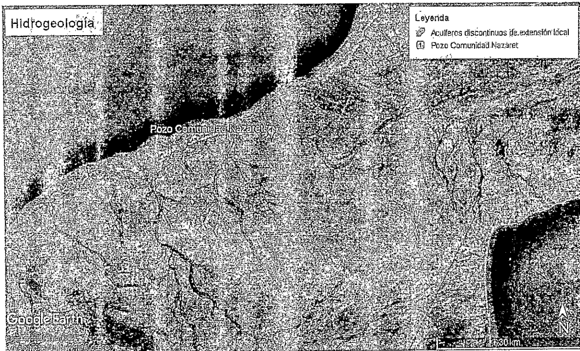
Figura 3. Hidrogeología
