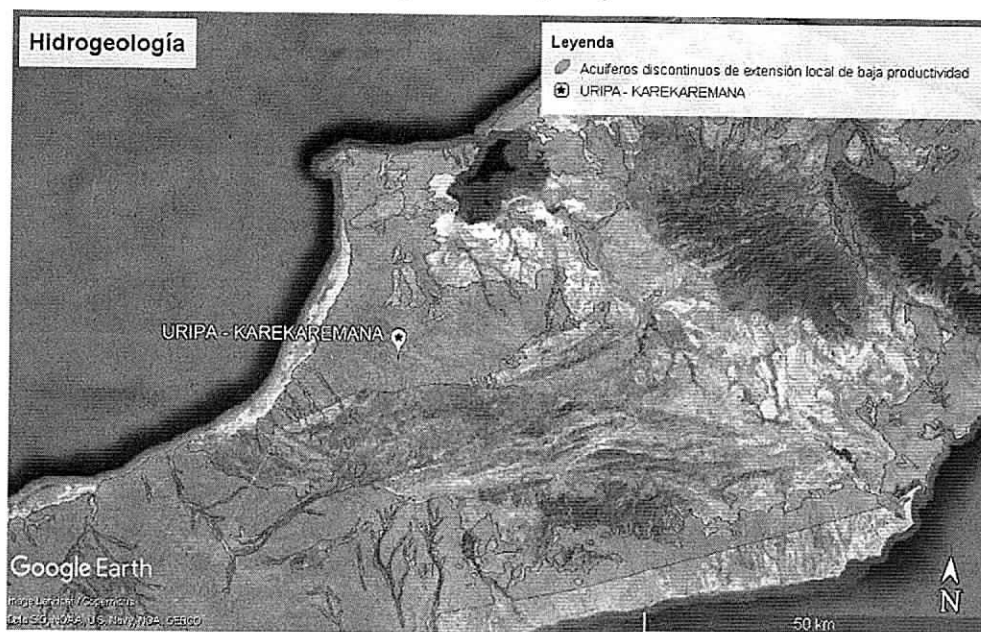
Figura 3. Hidrogeología
