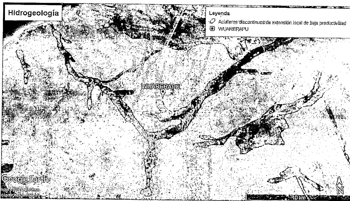
Figura 3. Hidrogeología
