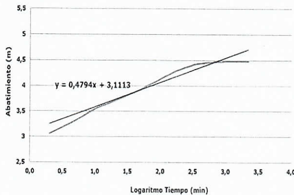
GRÁFICA PRUEBA DE RECUPERACIÓN - PZ No. 4 FINCA VILLA ARIAS - PORCIOSA - ALBANIA
