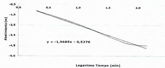
GRÁFICA PRUEBA DE RECUPERACIÓN - PZ No. 4 FINCA VILLA ARIAS - PORCIOSA - ALBANIA
