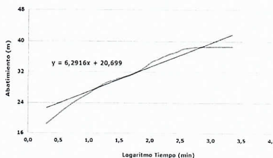
GRÁFICA DE LA PRUEBA DE BOMBEO - PZ No. 2 FINCA BUENOS AIRES - PORCIOSA - ALBANIA
