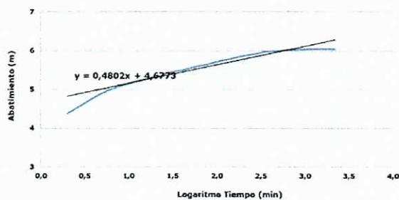
GRÁFICA PRUEBA DE RECUPERACIÓN - PZ No. 5 FINCA LAS MARGARITAS - PORCOSA - ALBANIA
