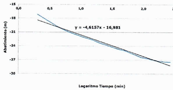
GRÁFICA PRUEBA DE RECUPERACIÓN - PZ No. 8 FINCA LOS DELIRIOS - PORCOSA - ALBANIA
