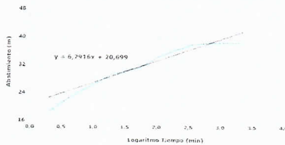
GRÁFICA DE LA PRUEBA DE BOMBEO - PZ No. 2 FINCA BUENOS AIRES - PORCIOSA - ALBANIA
