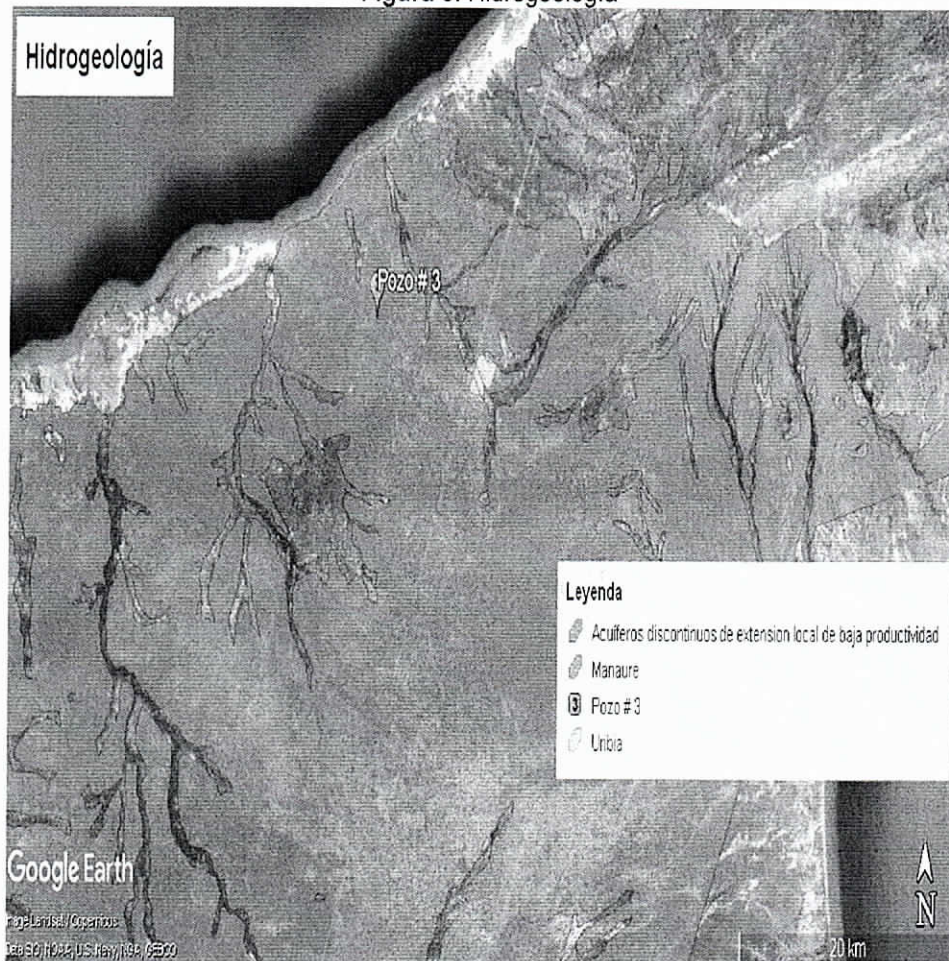
Figura 3. Hidrogeología
