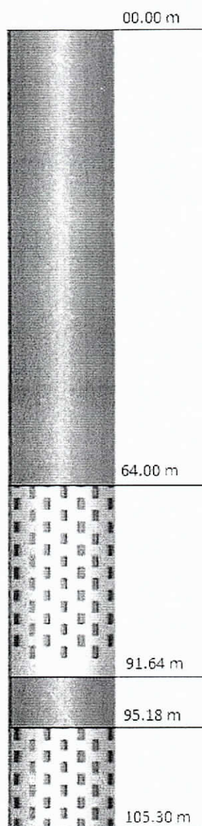
Figura 4. Diseño del pozo N° 3
