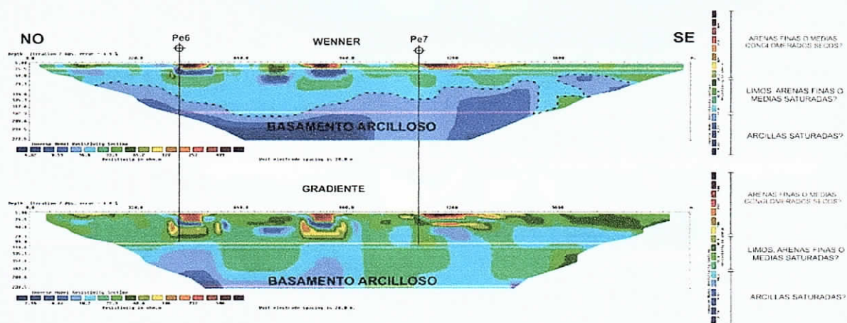
Figura 6. Modelo de resistividad T3.
