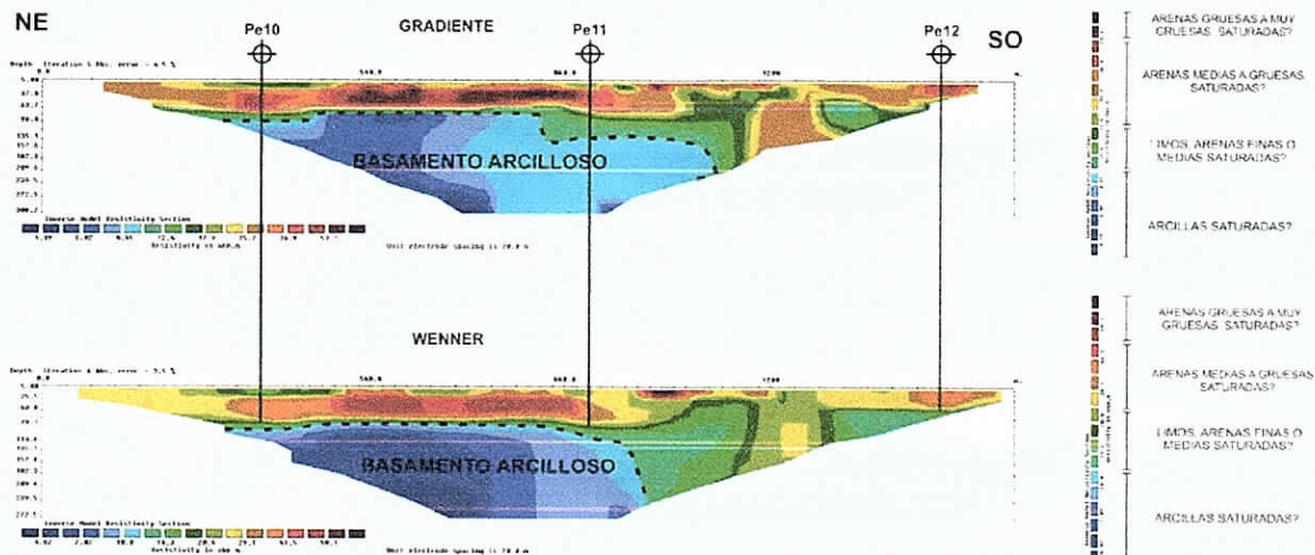
Figura 8. Modelo de resistividad T5.
