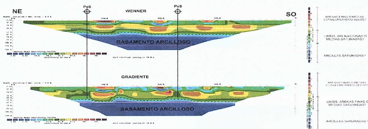
Figura 7. Modelo de resistividad T4.
