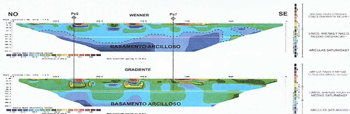
Figura 6. Modelo de resistividad T3.
