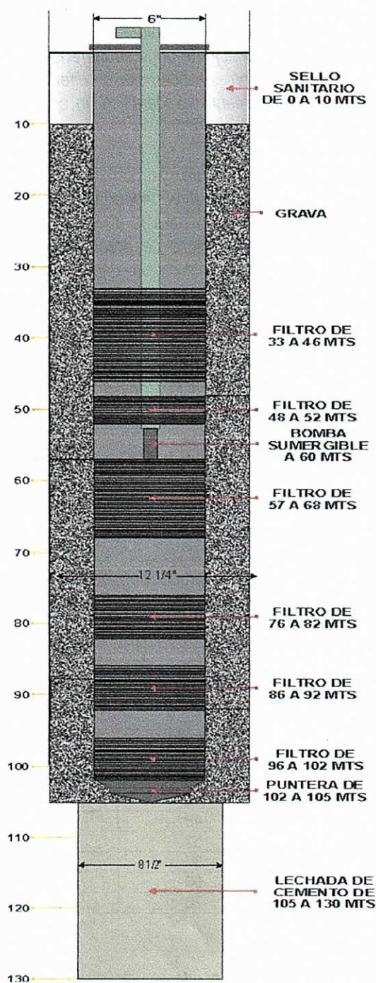
Figura 4. Diseño mecánico del pozo
