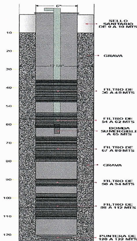
Figura 4. Diseño mecánico del pozo
