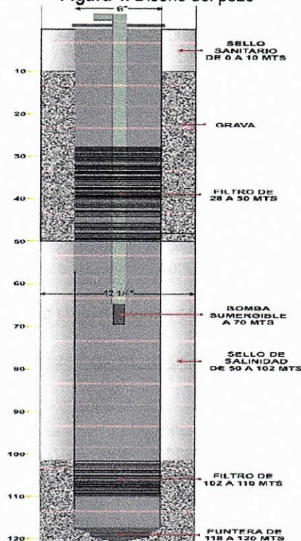
Figura 4. Diseño del pozo
