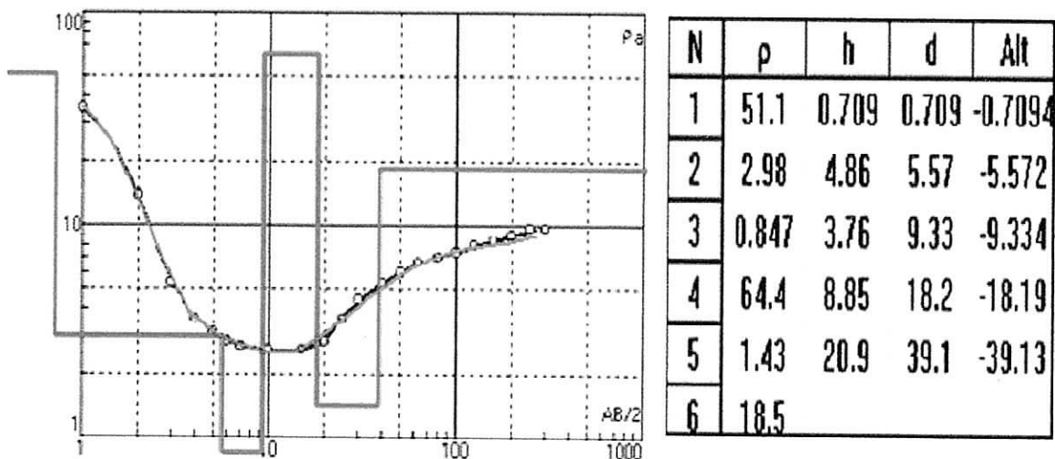
Figura 4. Curva teórica y modelación para el sondeo SEV01.
