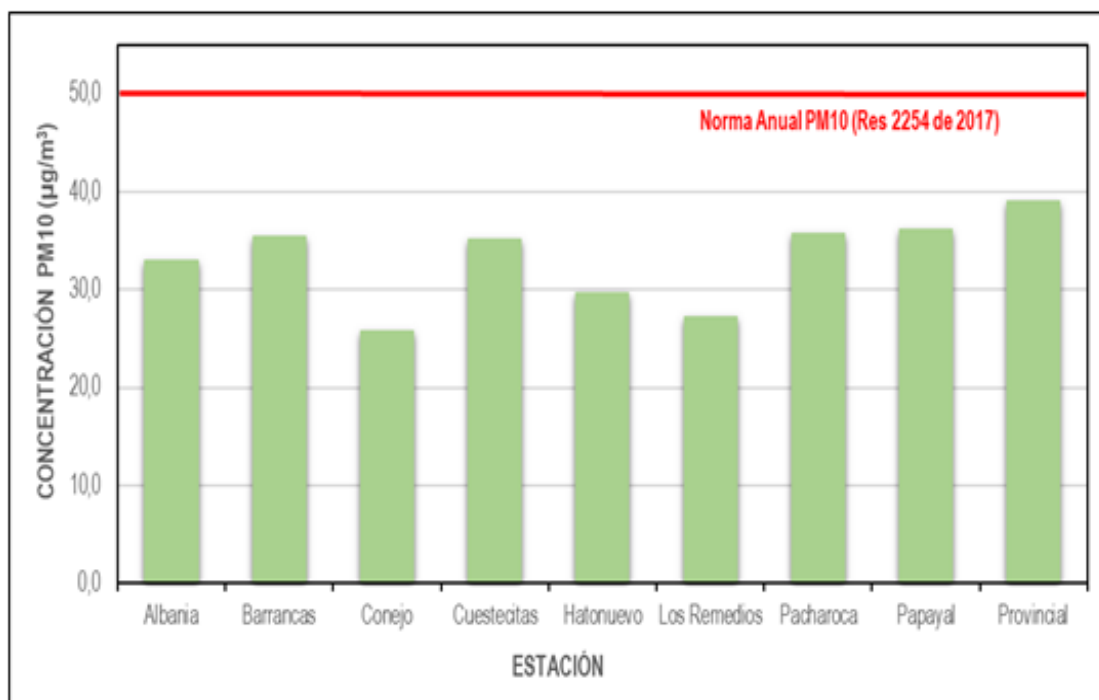
Figura 4. Promedio anual indicativo de PM10 para el 2019 en el SEVCA.
