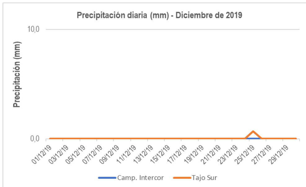
Figura 7. Precipitación diaria en diciembre de 2019.
