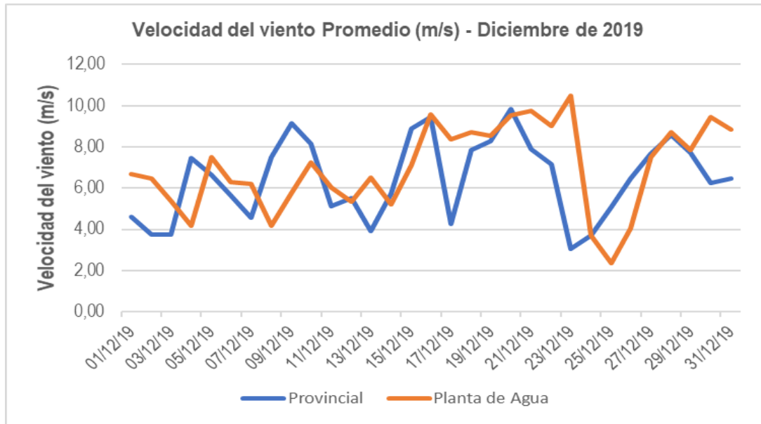
Figura 6. Comportamiento de la velocidad del viento diaria en diciembre de 2019.
