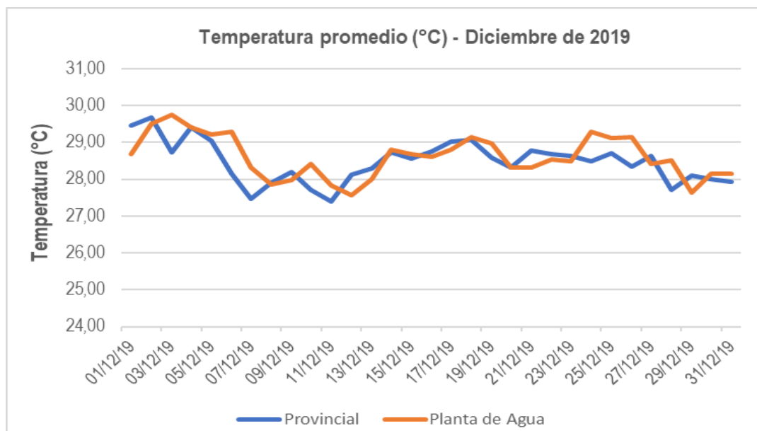
Figura 5. Comportamiento de la temperatura ambiente en diciembre de 2019.
