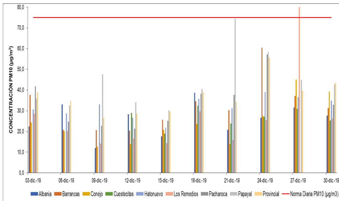
Figura 3. Comportamiento diario del PM10 en diciembre de 2019.
