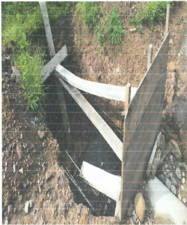
Imagen 5. Sitio intervenido ocupación de cauce punto 4, Box's Culverts
