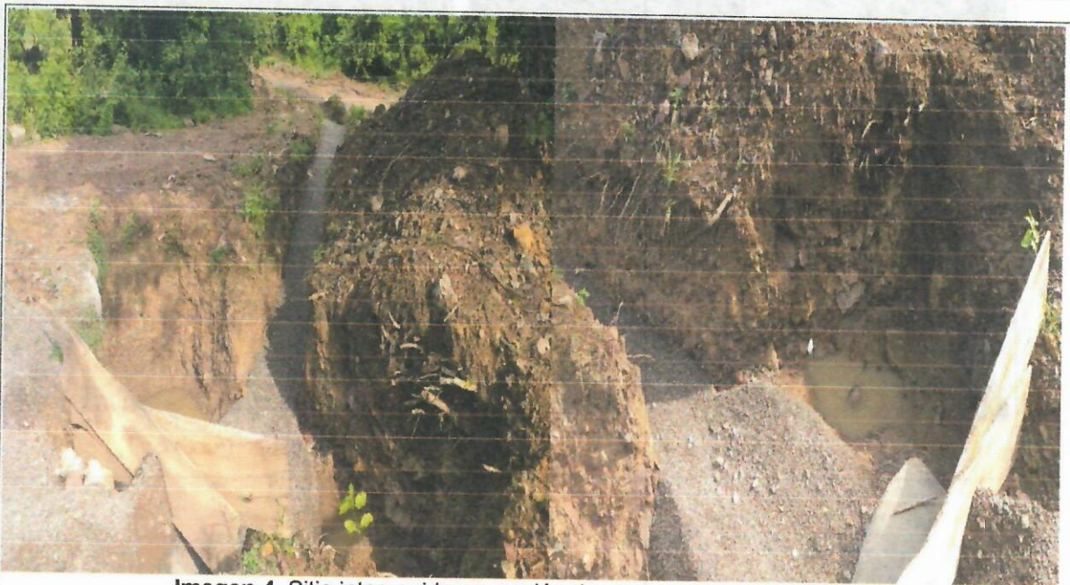
Imagen 4. Sitio intervenido ocupación de cauce punto 3, Box's Culverts
