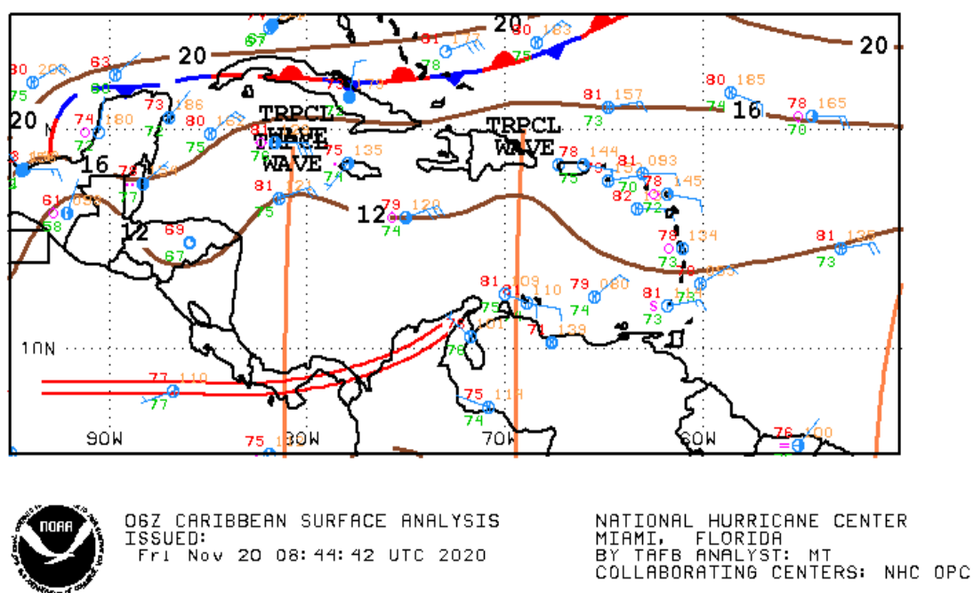
Figura 3: Muestra la ubicación de ondas tropicales en el Océano Atlántico y Mar Caribe, noviembre 20 de 2020. Fuente: NOAA
