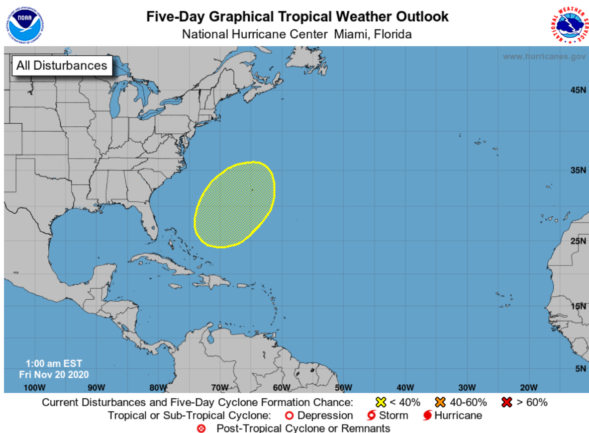
Figura 2: Proyección a 5 días de la situación meteorológica en el Mar Caribe. Fuente: NOAA.
