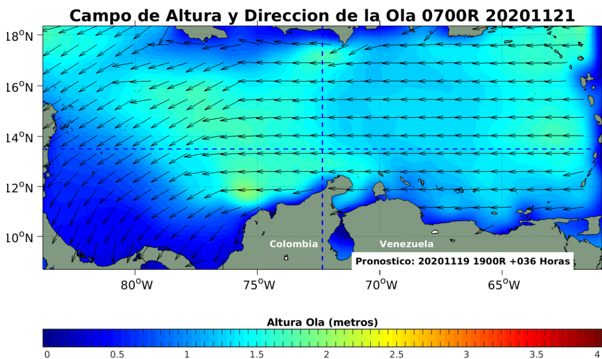
Figura 6: Pronóstico de la altura y dirección de las olas en el Mar Caribe, noviembre 20 de 2020. Fuente: CIOH.
