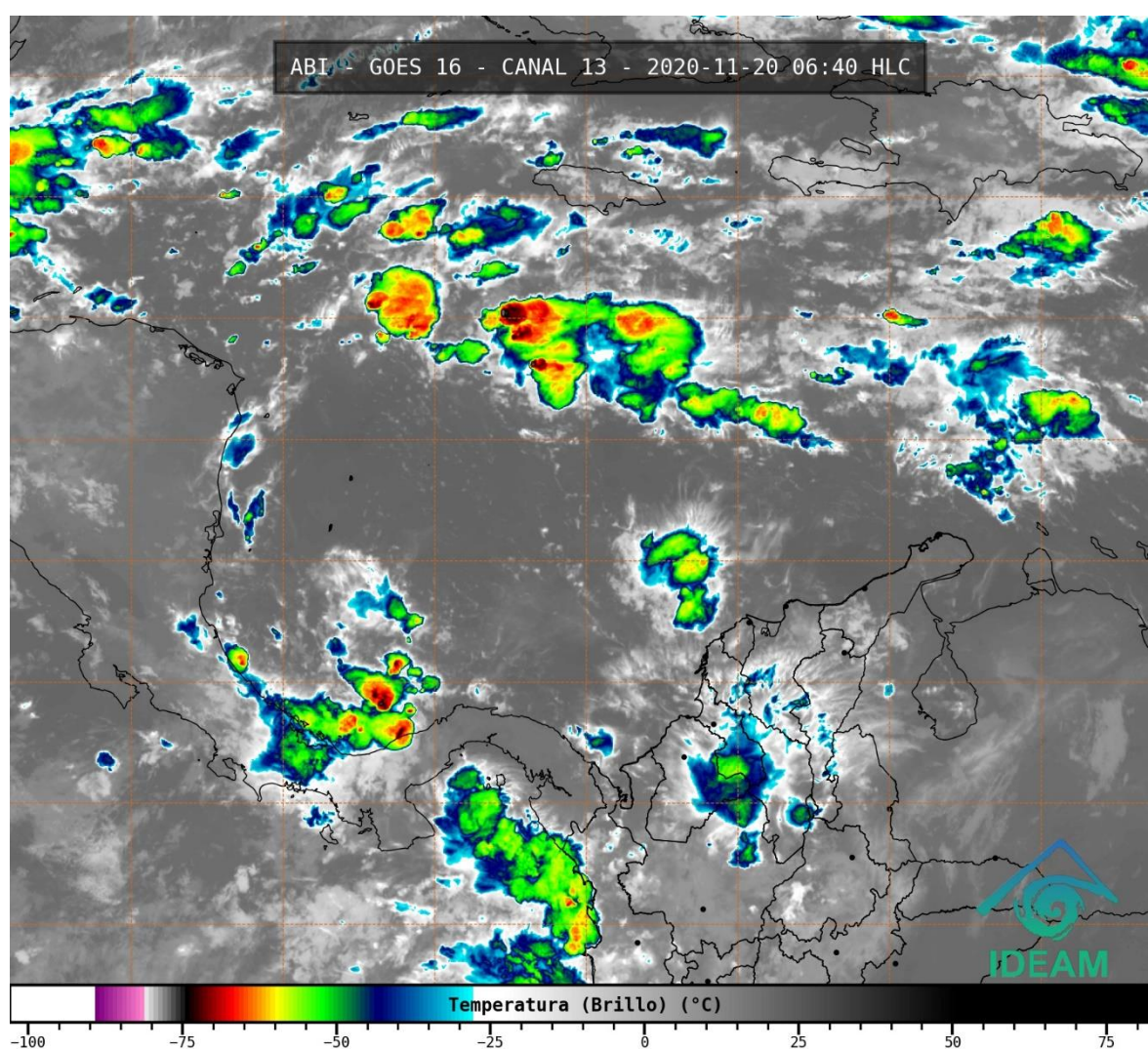
Figura 4: Imagen satelital GOES, noviembre 20 de 2020, hora 6:40 am de Colombia. Fuente: IDEAM
