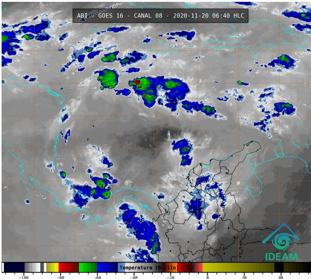
Figura 5: Imagen satelital GOES vapor de agua, noviembre 20 de 2020, hora 6:40 am de Colombia. Fuente: IDEAM.
