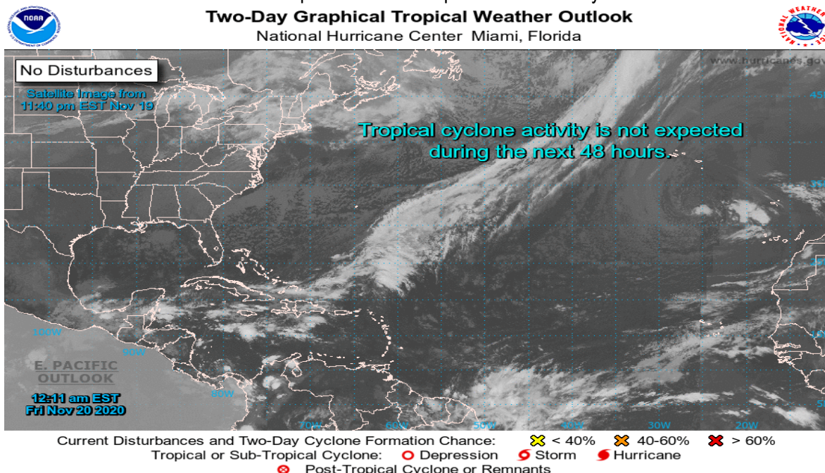
Figura 1: Situación meteorológica actual en el Mar Caribe, noviembre 20 de 2020, Fuente: NHC-NOAA.
