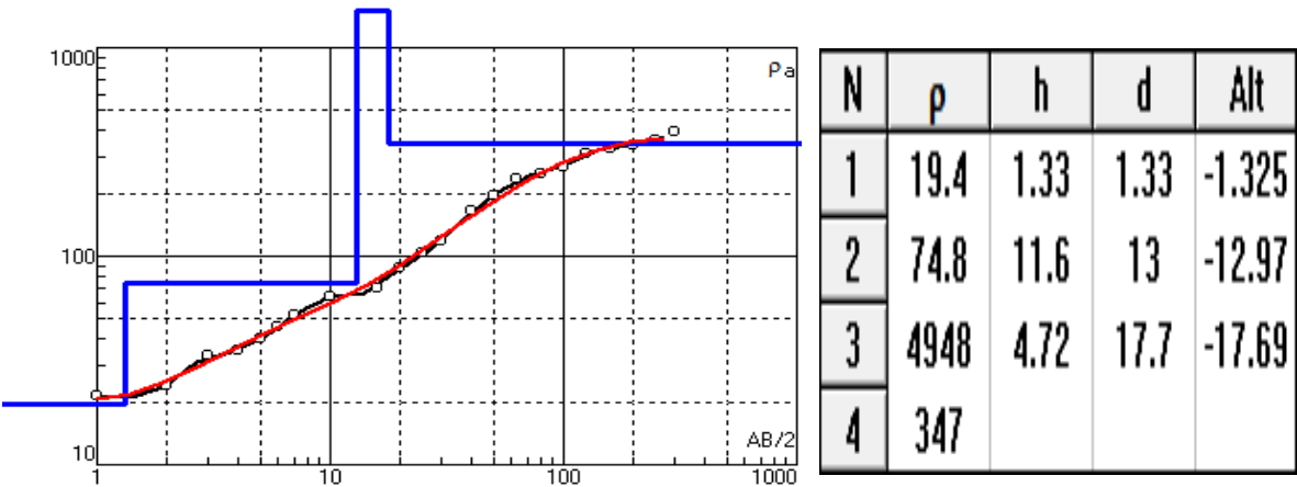
Figura 4. Curva teórica y modelación para el sondeo SEV
