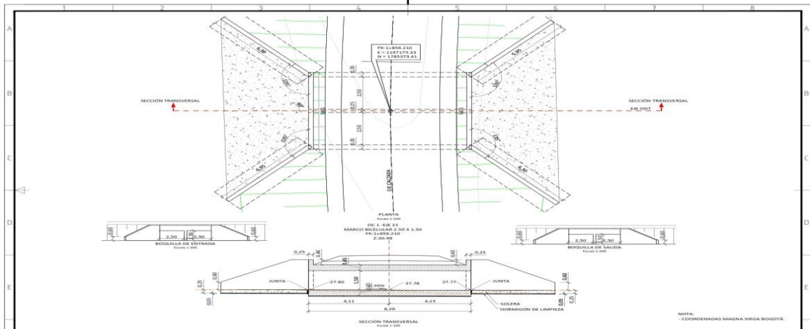
Grafica 7. Esquema de diseño de obras de arte proyectadas
