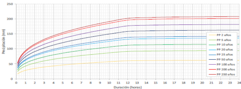
Grafica 5. Hidrograma de precipitación en la zona, fuente Estudio Hidráulico de la planta eólica Windpeshi (19516-04-04-IIH-ITE-001)
