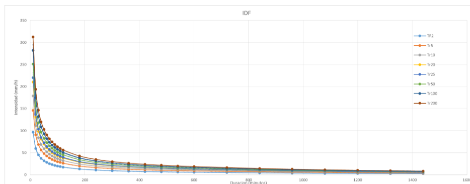
Grafica 6. Hidrógrafa intensidad lluvias por eventos
