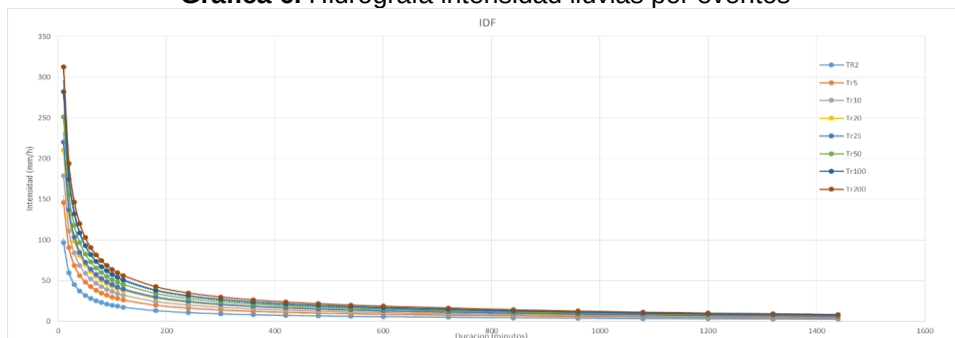
Grafica 6. Hidrógrafa intensidad lluvias por eventos
