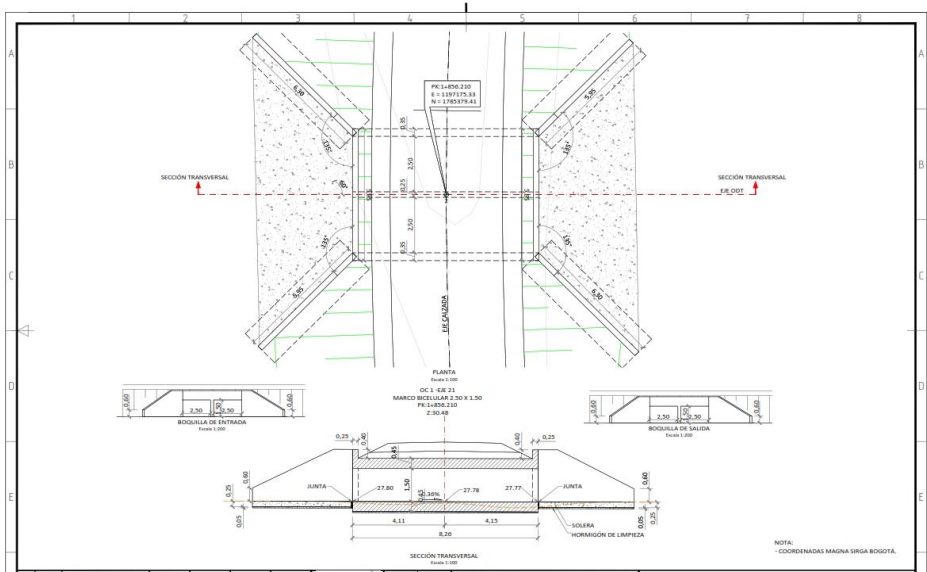
Figura 7. Esquema de diseño de obras de arte proyectadas
