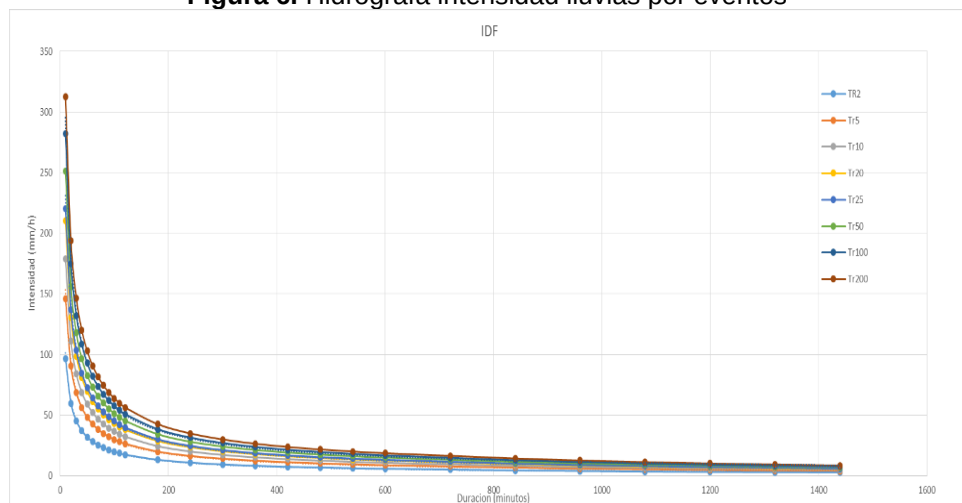
Figura 6. Hidrógrafa intensidad lluvias por eventos
