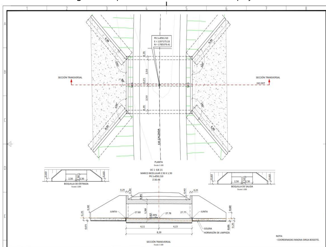
Figura 7. Esquema de diseño de obras de arte proyectadas
