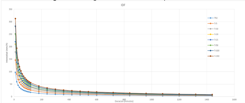
Figura 6. Hidrógrafa intensidad lluvias por eventos
