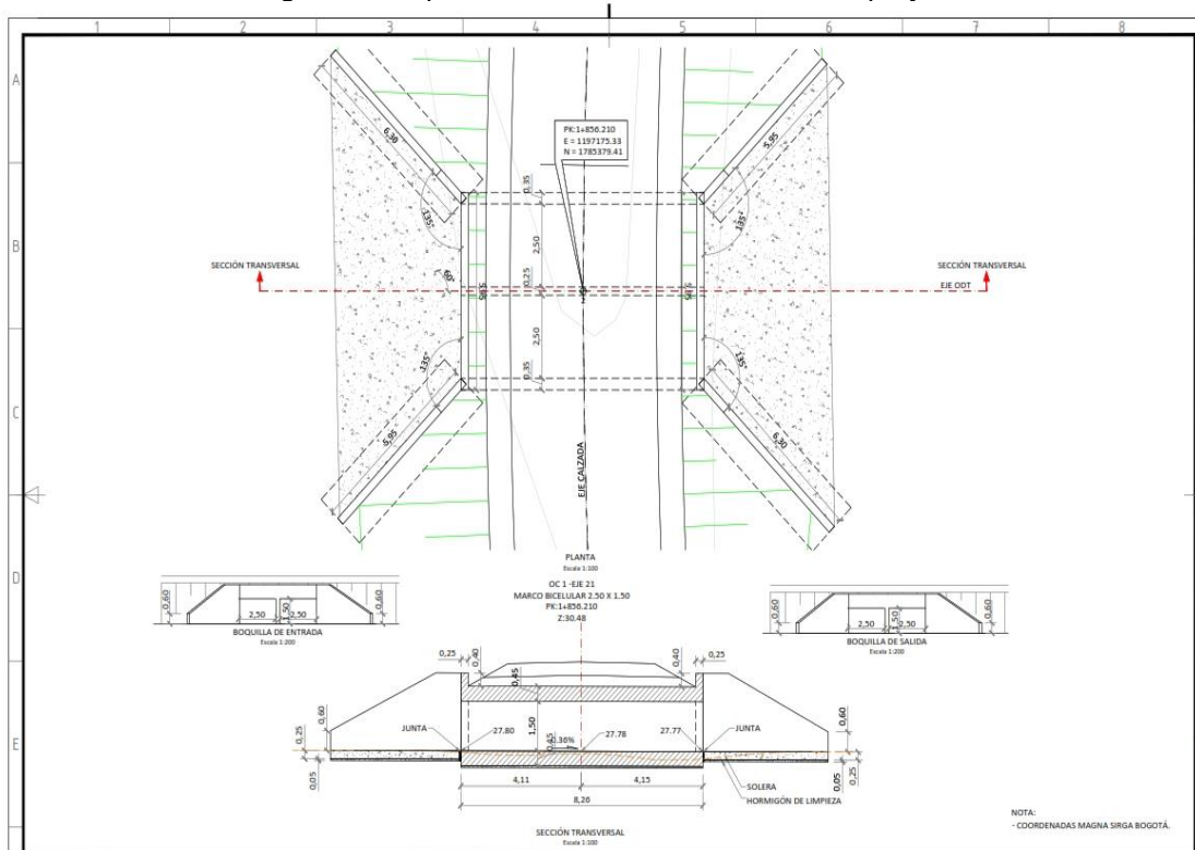
Figura 7. Esquema de diseño de obras de arte proyectadas
