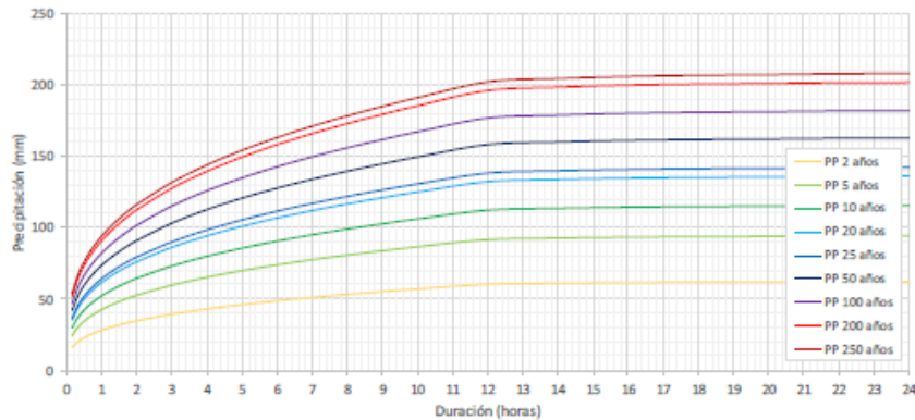
Figura 5. Hidrograma de precipitación en la zona, fuente Estudio Hidráulico de la planta eólica Windpeshi (19516-04-04-IIH-ITE-001)
