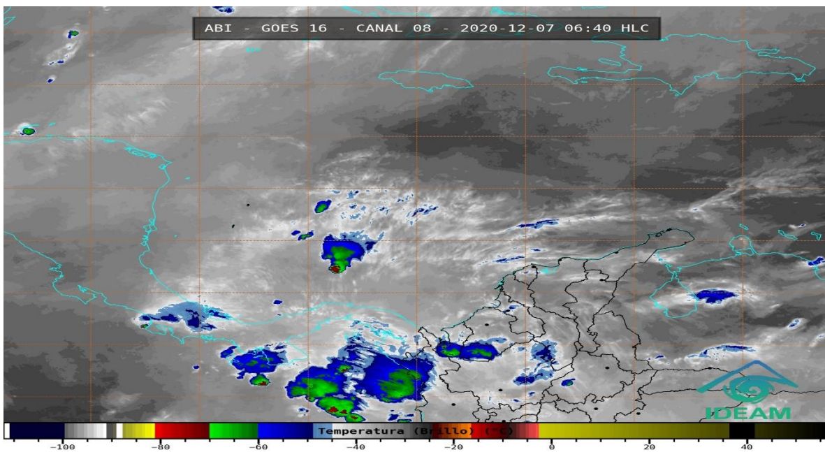
Figura 5: Imagen satelital GOES vapor de agua, diciembre 7 de 2020, hora 6:40 am de Colombia. Fuente: IDEAM.
