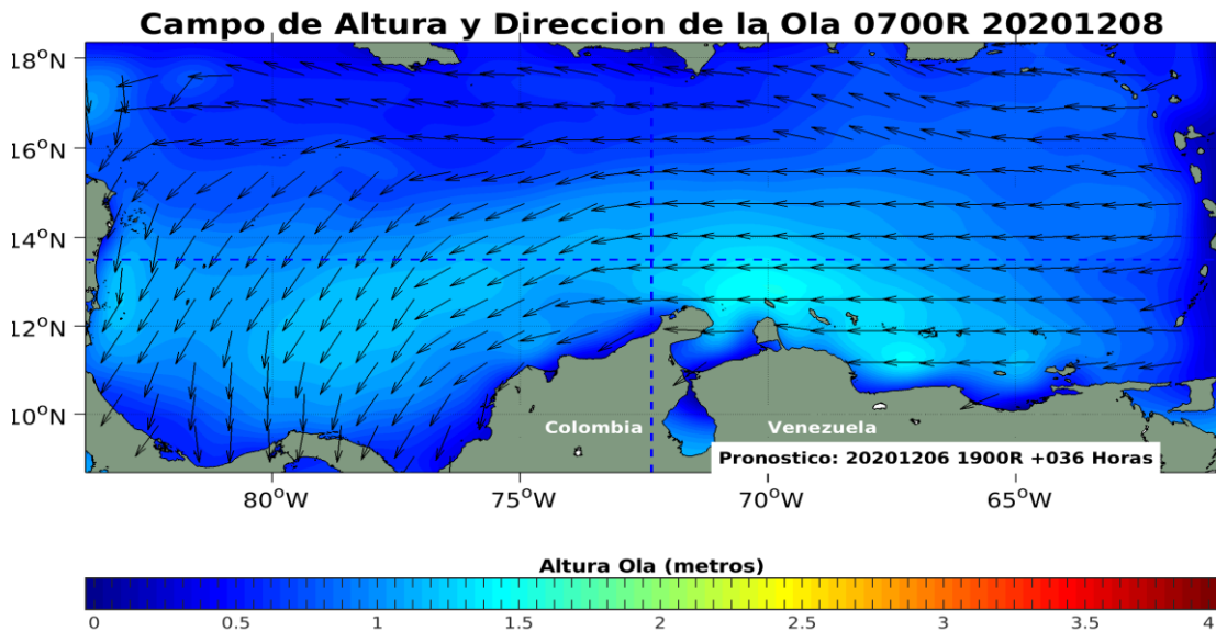
Figura 6: Pronóstico de la altura y dirección de las olas en el Mar Caribe, diciembre 7 de 2020. Fuente: CIOH.
