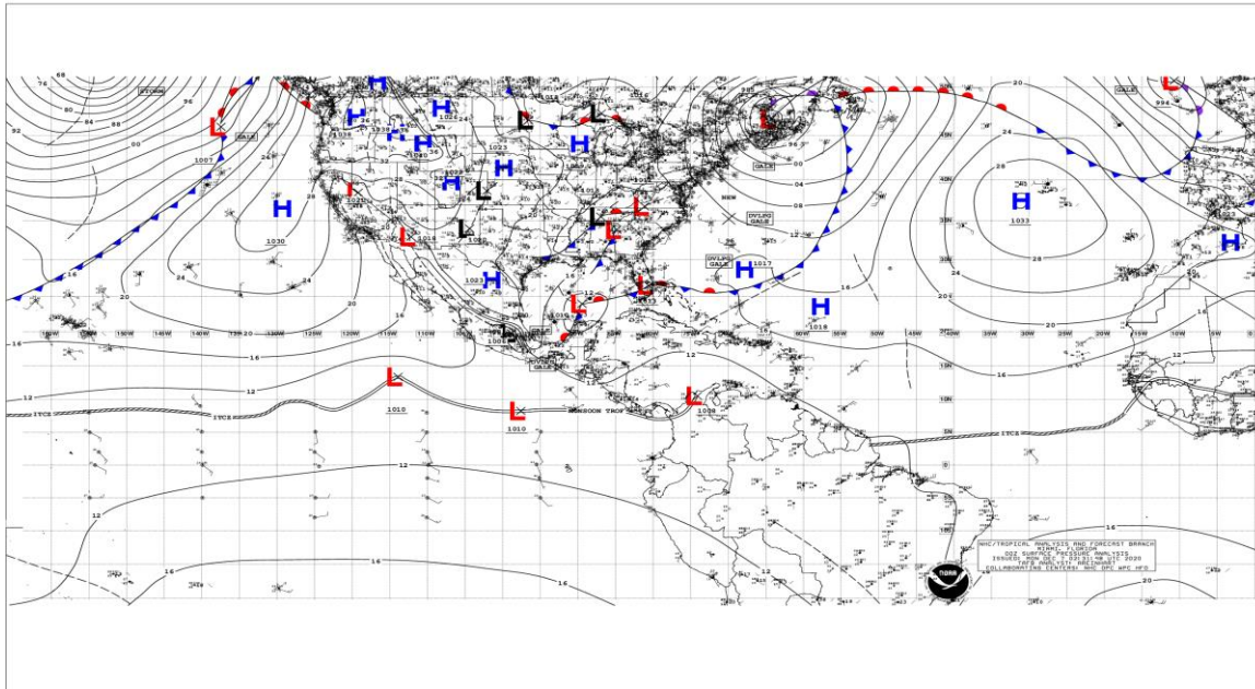
Figura 1: Situación meteorológica actual en el Mar Caribe y Océano Atlántico, diciembre 7 de 2020, Fuente: NHC NOAA.
