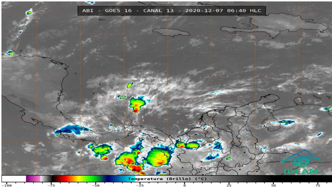
Figura 4: Imagen satelital GOES, diciembre 7 de 2020, hora 6:40 am de Colombia. Fuente: NOAA.
