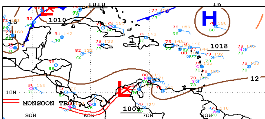
Figura 1: Situación meteorológica actual en el Mar Caribe y Océano Atlántico, diciembre 7 de 2020, Fuente: NHC NOAA.
