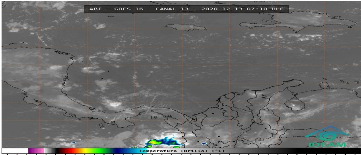
Figura 4: Imagen satelital GOES, diciembre 13 de 2020, hora 7:10 am de Colombia. Fuente: IDEAM
