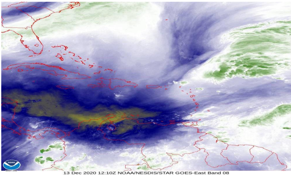
Figura 5: Imagen satelital GOES vapor de agua, diciembre 13 de 2020, hora 7:10 am de Colombia. Fuente: NOAA.
