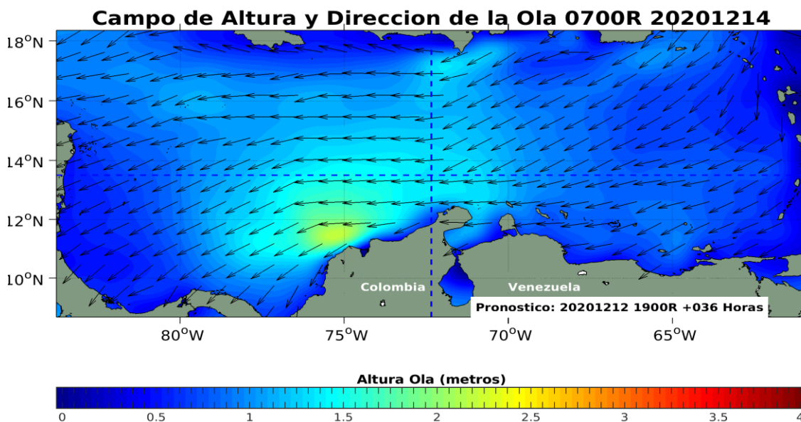
Figura 6: Pronóstico de la altura y dirección de las olas en el Mar Caribe, diciembre 13 de 2020. Fuente: CIOH.
