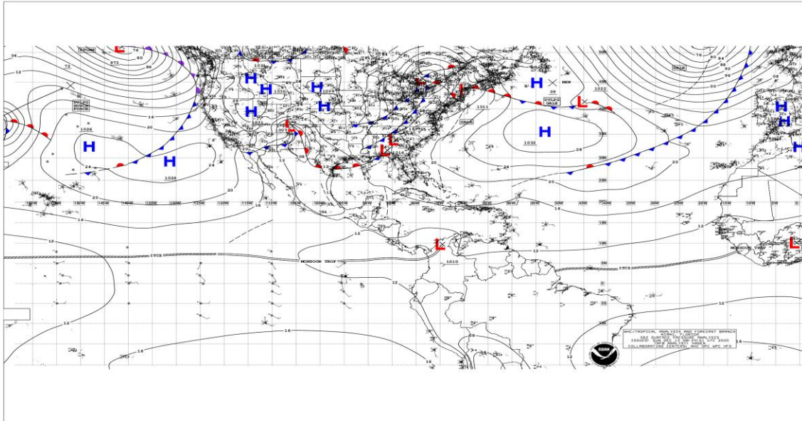
Figura 1: Situación meteorológica actual en el Mar Caribe y Océano Atlántico, diciembre 13 de 2020, Fuente: NHC NOAA.
