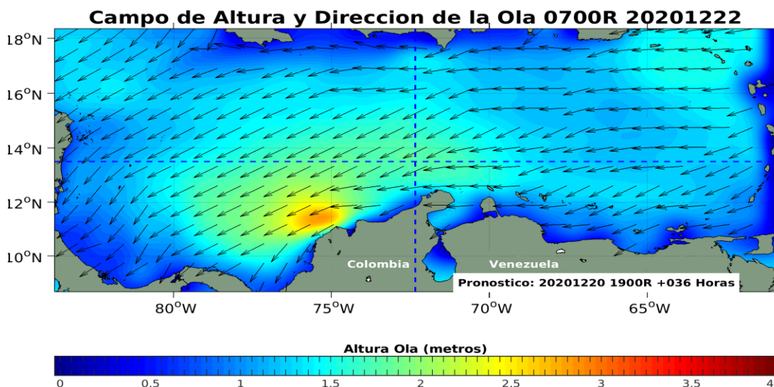
Figura 6: Pronóstico de la altura y dirección de las olas en el Mar Caribe, diciembre 21 de 2020. Fuente: CIOH.
