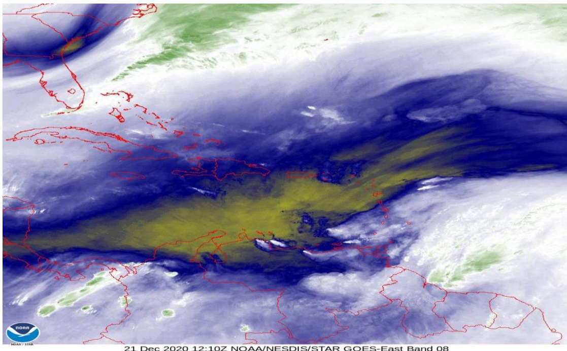
Figura 5: Imagen satelital GOES vapor de agua, diciembre 21 de 2020, hora 7:10 am de Colombia. Fuente: NOAA.
