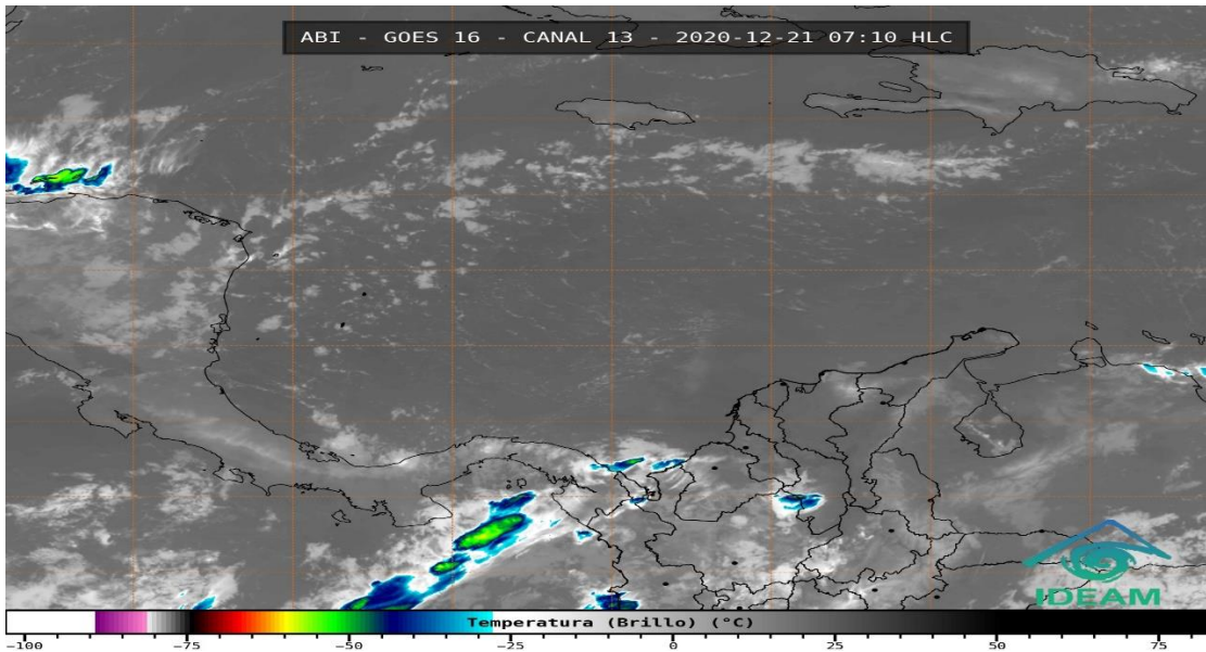
Figura 4: Imagen satelital GOES, diciembre 21 de 2020, hora 7:10 am de Colombia. Fuente: IDEAM
