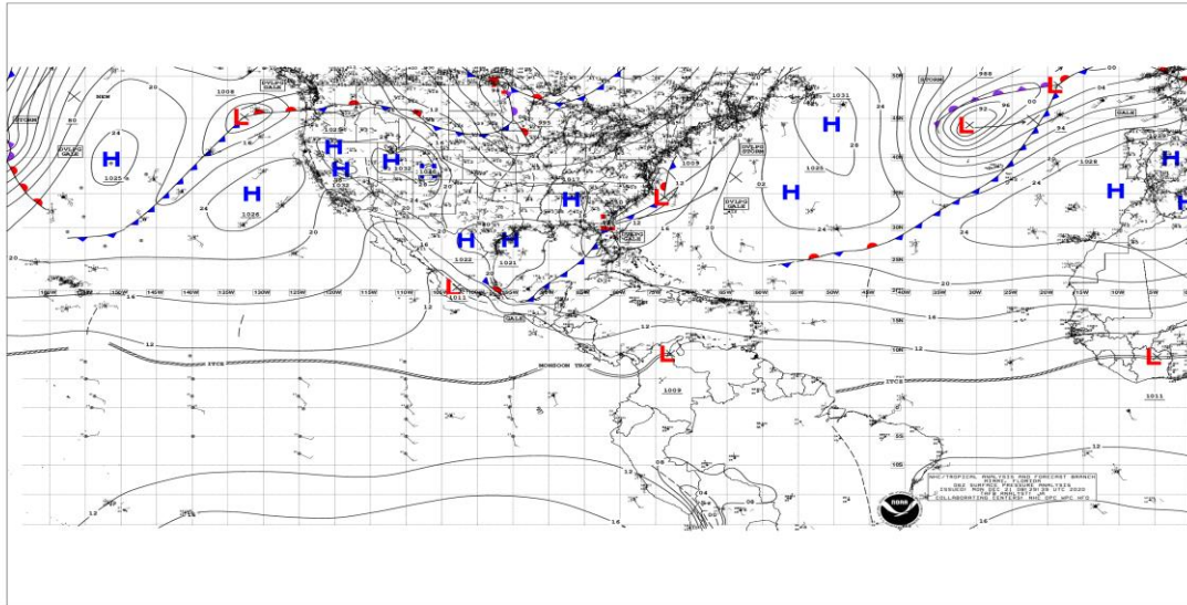
Figura 1: Situación meteorológica actual en el Mar Caribe y Océano Atlántico, diciembre 21 de 2020, Fuente: NHC NOAA.
