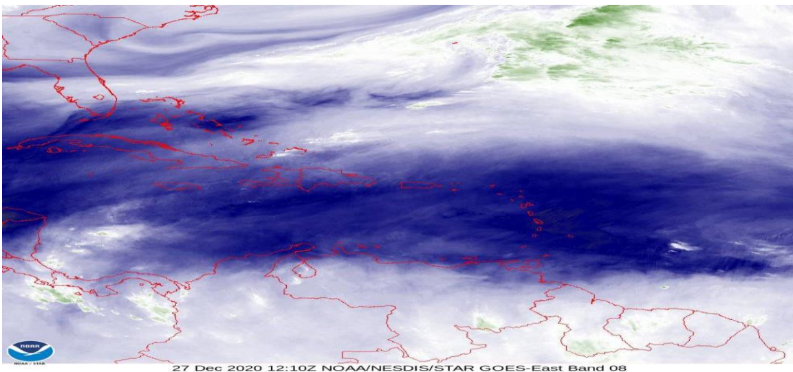
Figura 5: Imagen satelital GOES vapor de agua, diciembre 27 de 2020, hora 7:10 am de Colombia. Fuente: NOAA.
