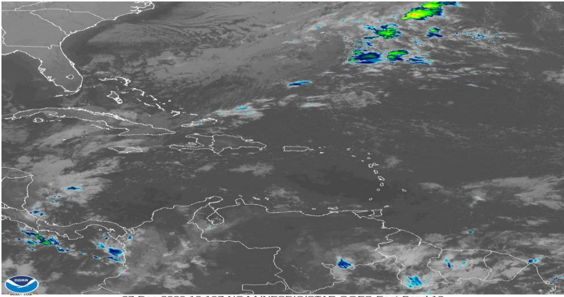
Figura 4: Imagen satelital GOES, diciembre 27 de 2020, hora 7:10 am de Colombia. Fuente: NOAA
