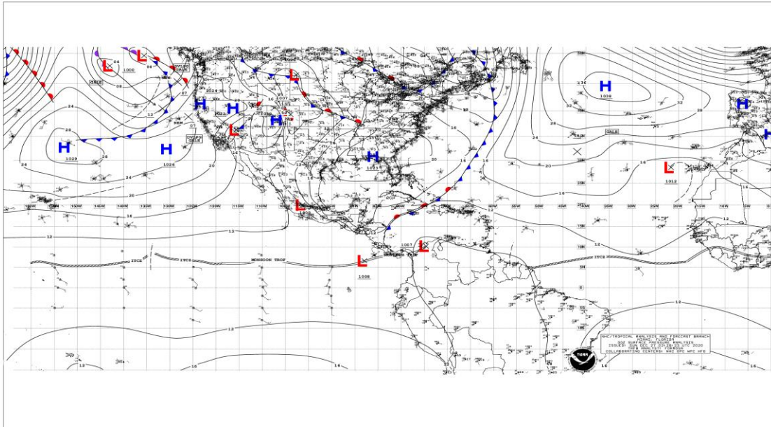
Figura 1: Situación meteorológica actual en el Mar Caribe y Océano Atlántico, diciembre 27 de 2020, Fuente: NHC NOAA.
