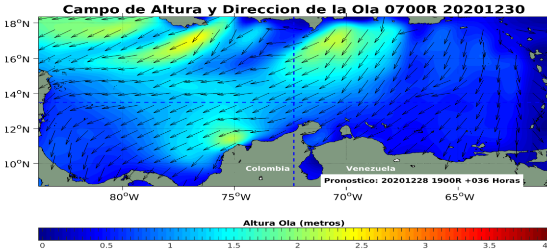
Figura 6: Pronóstico de la altura y dirección de las olas en el Mar Caribe, diciembre 29 de 2020. Fuente: CIOH.
