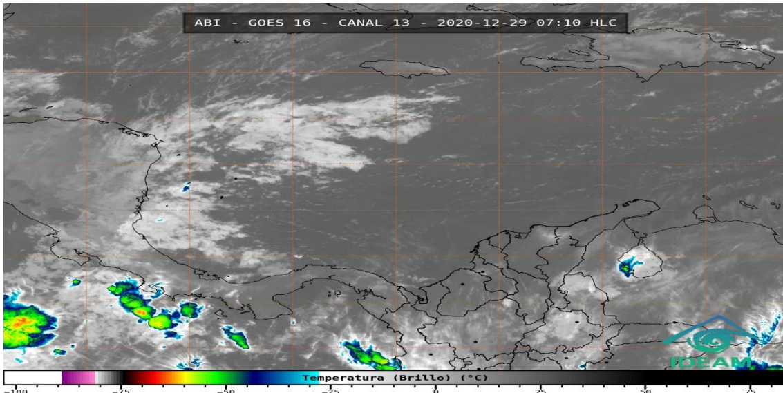
Figura 4: Imagen satelital GOES, diciembre 29 de 2020, hora 7:10 am de Colombia. Fuente: IDEAM
