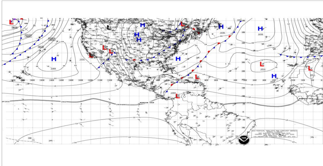
Figura 1: Situación meteorológica actual en el Mar Caribe y Océano Atlántico, diciembre 29 de 2020, Fuente: NHC NOAA.
