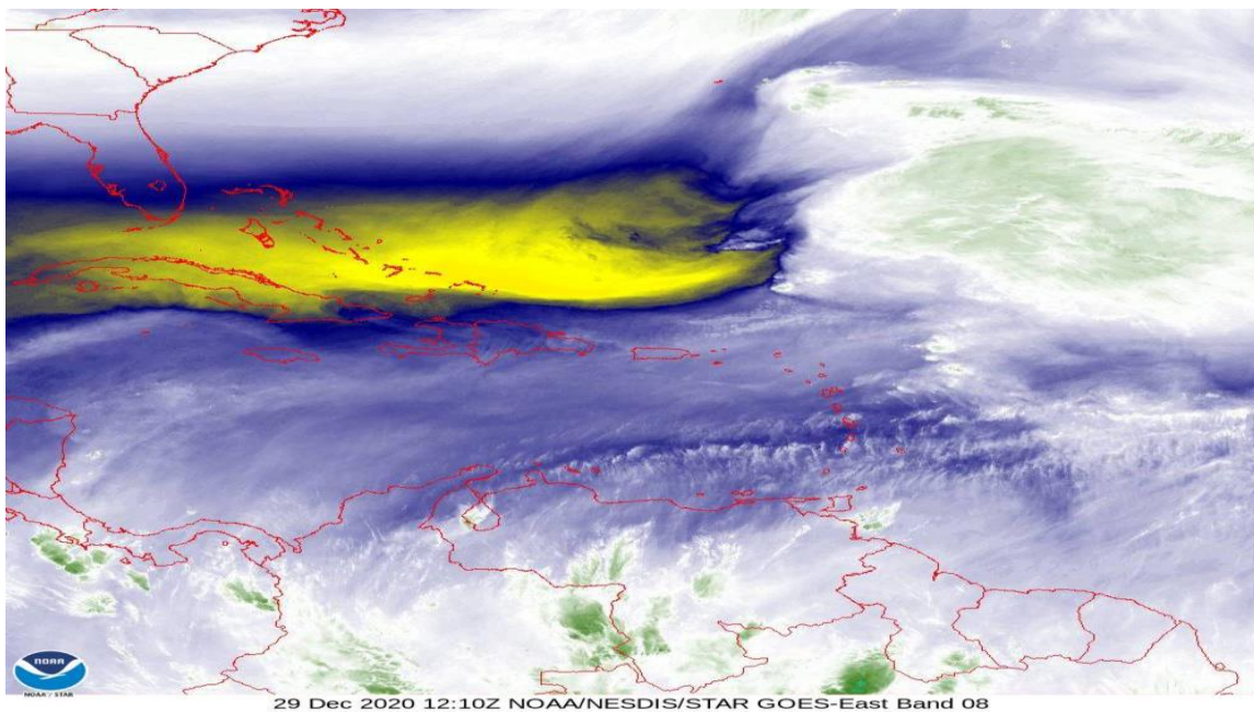
Figura 5: Imagen satelital GOES vapor de agua, diciembre 29 de 2020, hora 7:10 am de Colombia. Fuente: NOAA.
