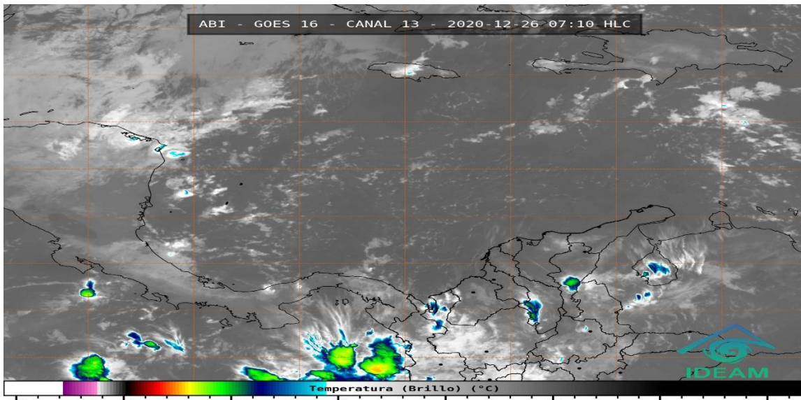
Figura 4: Imagen satelital GOES, diciembre 26 de 2020, hora 7:10 am de Colombia. Fuente: IDEAM
