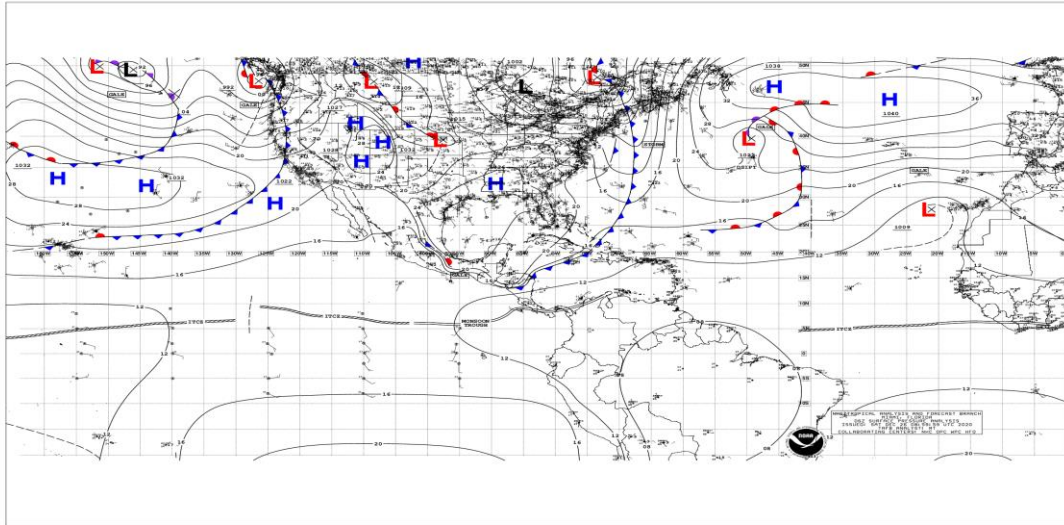
Figura 1: Situación meteorológica actual en el Mar Caribe y Océano Atlántico, diciembre 26 de 2020, Fuente: NHC NOAA.
