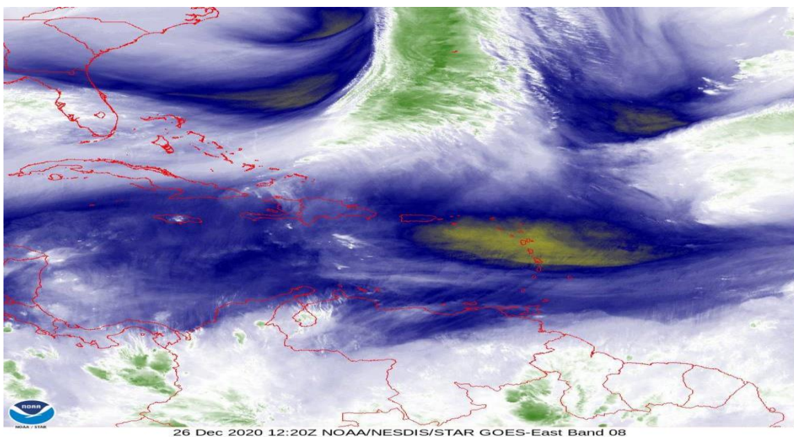
Figura 5: Imagen satelital GOES vapor de agua, diciembre 26 de 2020, hora 7:20 am de Colombia. Fuente: NOAA.
