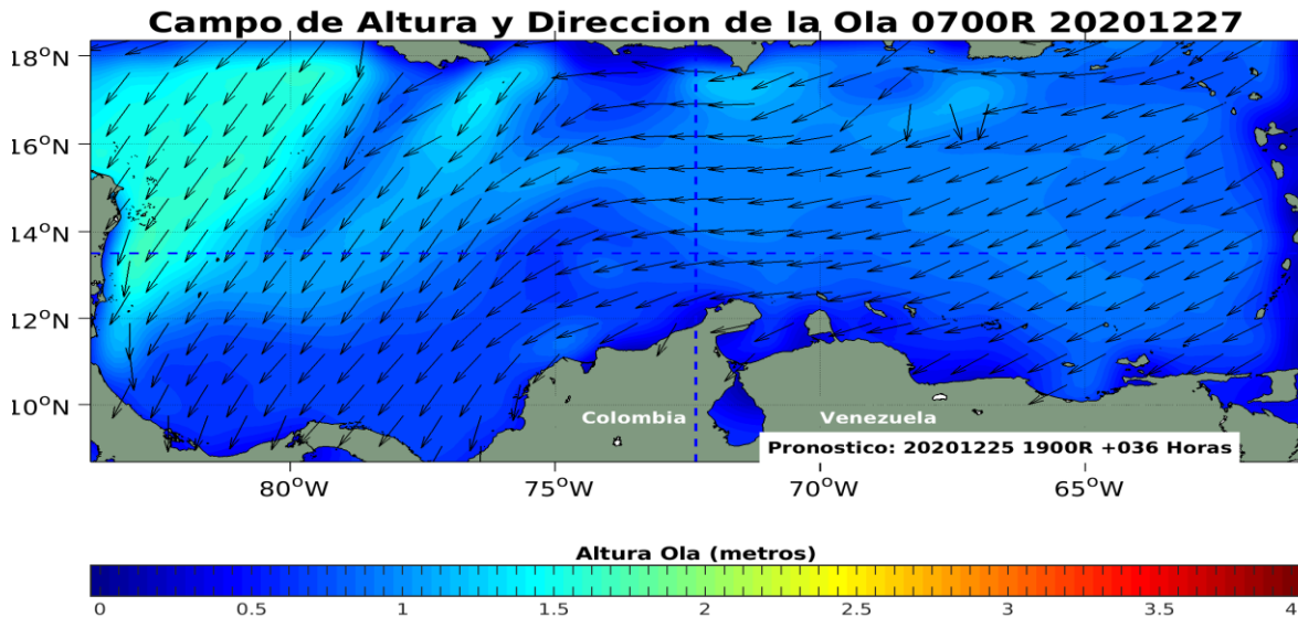
Figura 6: Pronóstico de la altura y dirección de las olas en el Mar Caribe, diciembre 26 de 2020. Fuente: CIOH.
