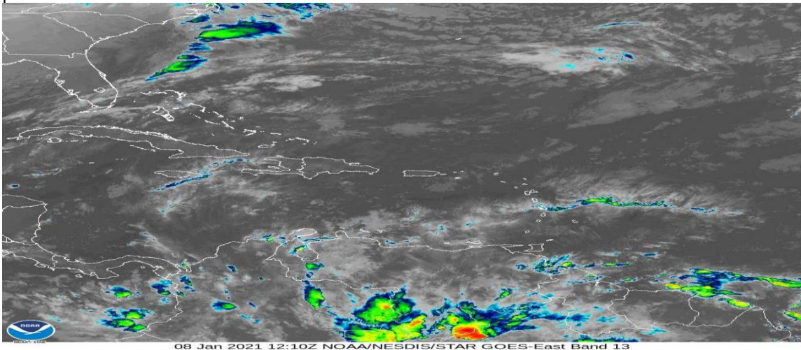
Figura 4: Imagen satelital GOES, enero 8 de 2021, hora 7:10 am de Colombia. Fuente: NOAA.
