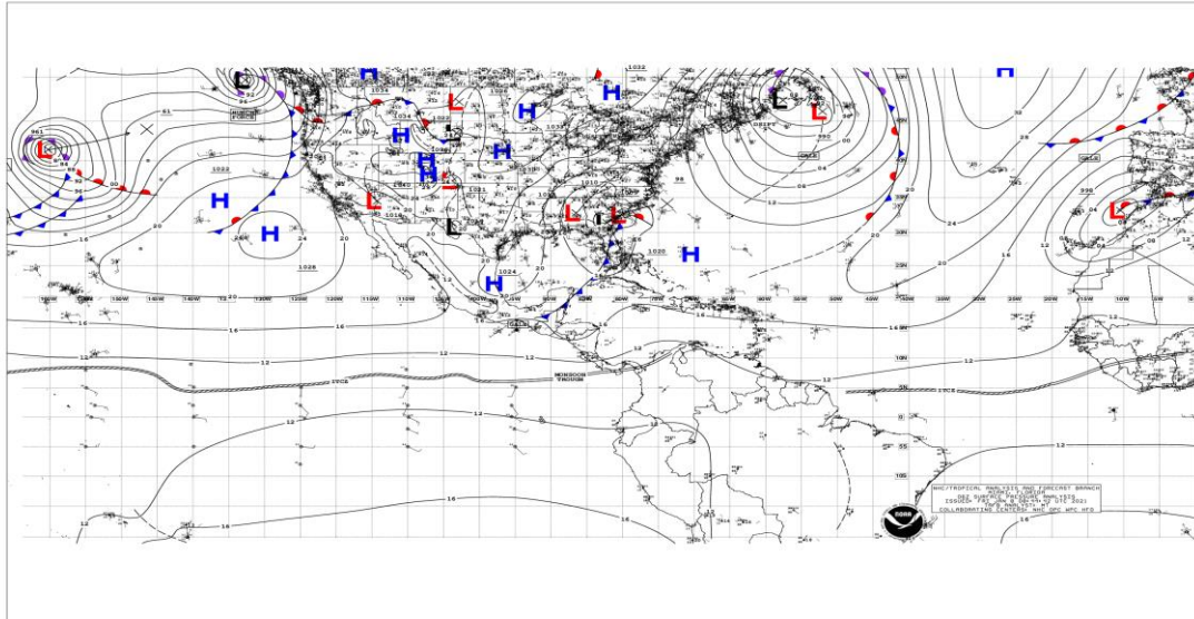
Figura 1: Situación meteorológica actual en el Mar Caribe y Océano Atlántico, enero 8 de 2021, Fuente: NHC NOAA.
