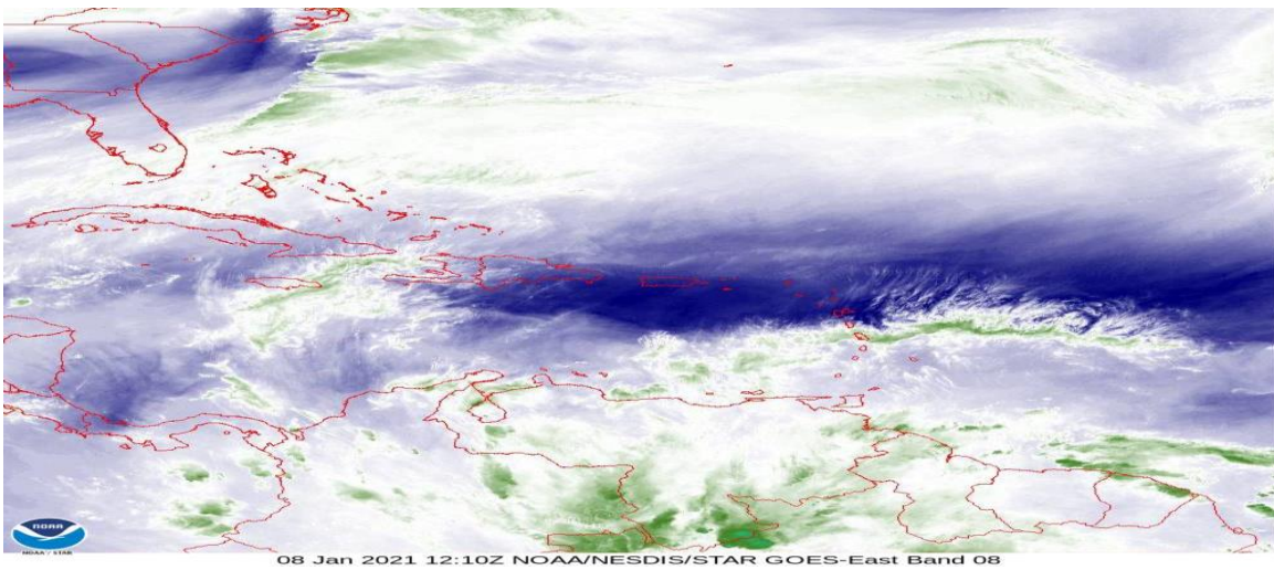
Figura 5: Imagen satelital GOES vapor de agua, enero 8 de 2021, hora 7:10 am de Colombia. Fuente: NOAA.
