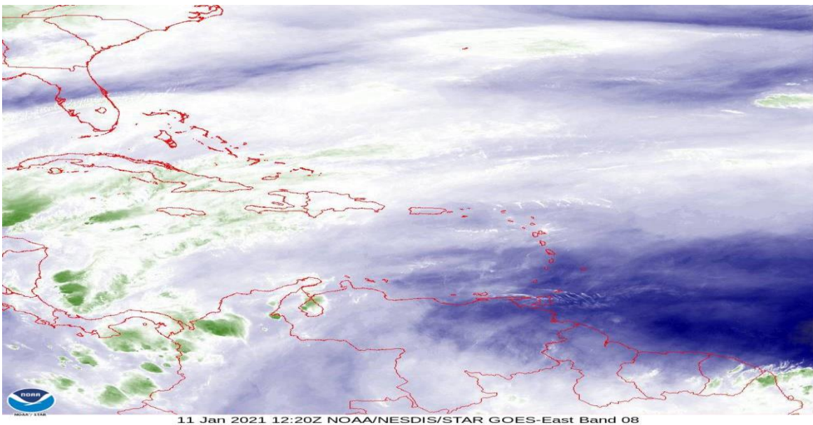
Figura 5: Imagen satelital GOES vapor de agua, enero 11 de 2021, hora 7:20 am de Colombia. Fuente: NOAA.
