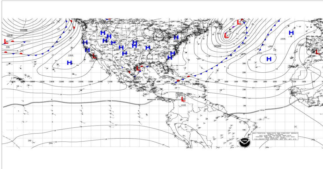
Figura 1: Situación meteorológica actual en el Mar Caribe y Océano Atlántico, enero 11 de 2021, Fuente: NHC NOAA.
