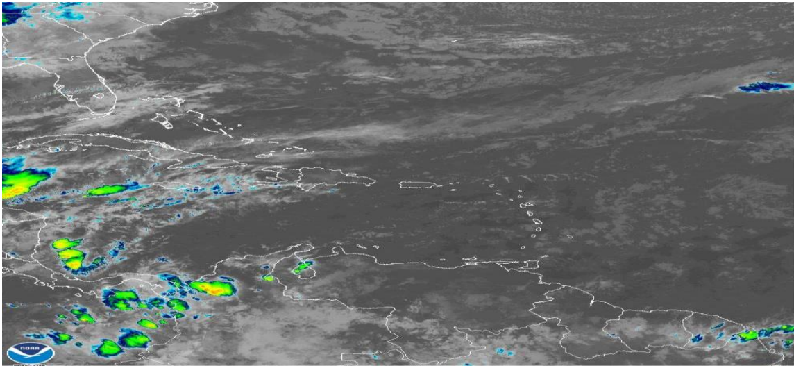
Figura 4: Imagen satelital GOES, enero 11 de 2021, hora 7:20 am de Colombia. Fuente: NOAA.
