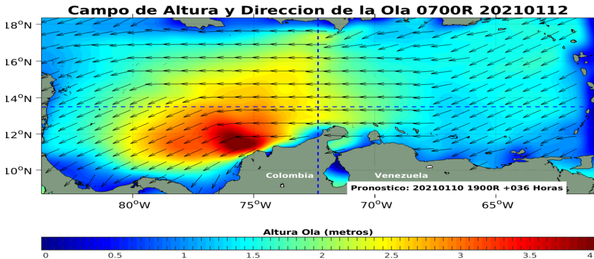
Figura 6: Pronóstico de la altura y dirección de las olas en el Mar Caribe, enero 11 de 2021. Fuente: CIOH.
