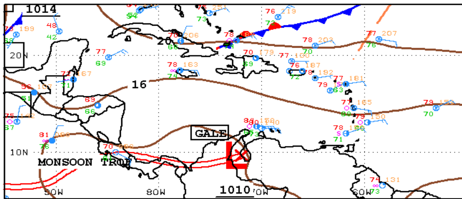
Figura 1: Situación meteorológica actual en el Mar Caribe y Océano Atlántico, enero 11 de 2021, Fuente: NHC NOAA.
