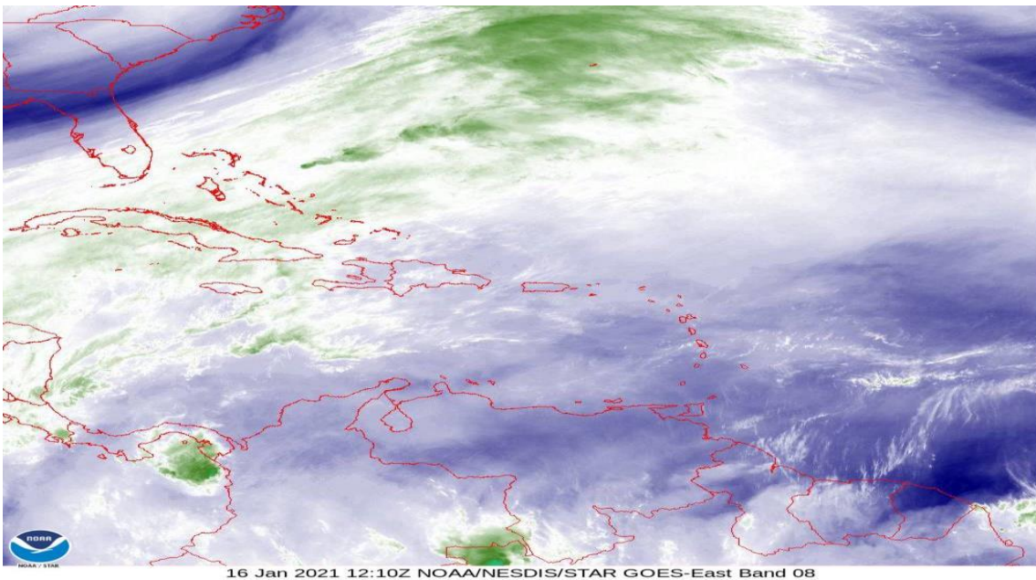
Figura 5: Imagen satelital GOES vapor de agua, enero 16 de 2021, hora 7:10 am de Colombia. Fuente: NOAA.
