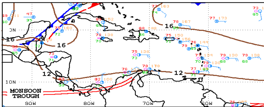
Figura 1: Situación meteorológica actual en el Mar Caribe y Océano Atlántico, enero 16 de 2021, Fuente: NHC NOAA.
