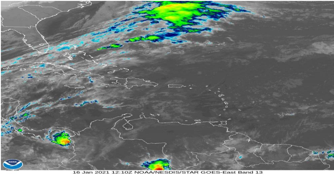
Figura 4: Imagen satelital GOES, enero 16 de 2021, hora 7:10 am de Colombia. Fuente: NOAA.
