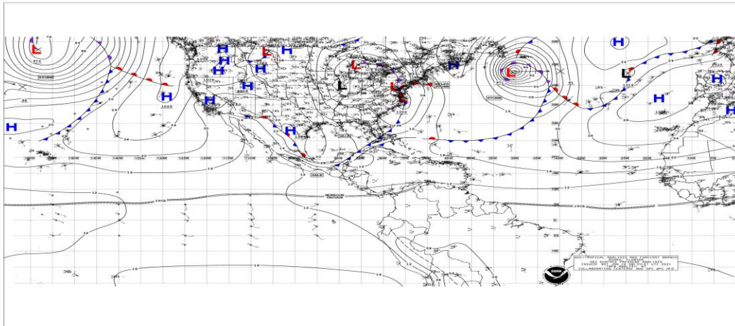
Figura 1: Situación meteorológica actual en el Mar Caribe y Océano Atlántico, enero 16 de 2021, Fuente: NHC NOAA.
