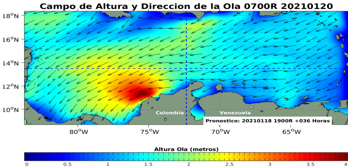
Figura 6: Pronóstico de la altura y dirección de las olas en el Mar Caribe, enero 19 de 2021. Fuente: CIOH.
