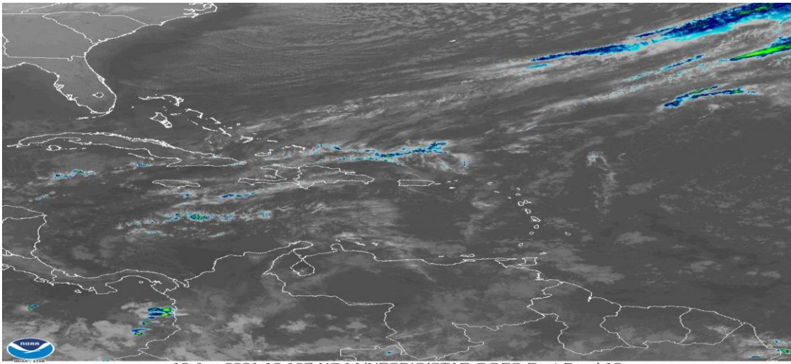
Figura 4: Imagen satelital GOES, enero 19 de 2021, hora 7:10 am de Colombia. Fuente: NOAA.
