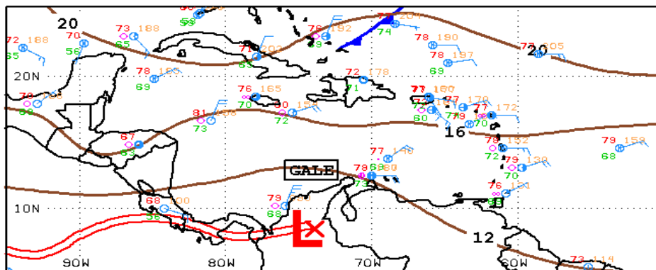
Figura 1: Situación meteorológica actual en el Mar Caribe y Océano Atlántico, enero 19 de 2021, Fuente: NHC NOAA.
