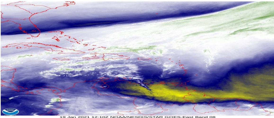
Figura 5: Imagen satelital GOES vapor de agua, enero 19 de 2021, hora 7:10 am de Colombia. Fuente: NOAA.
