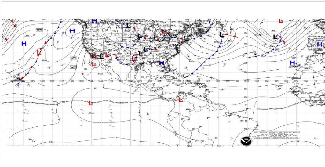
Figura 1: Situación meteorológica actual en el Mar Caribe y Océano Atlántico, enero 19 de 2021, Fuente: NHC NOAA.
