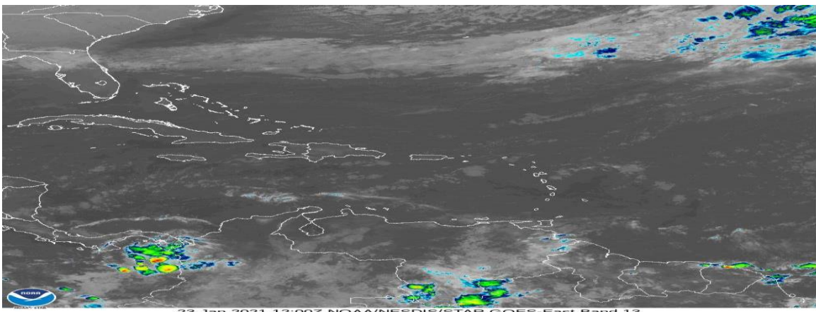
Figura 4: Imagen satelital GOES, enero 23 de 2021, hora 7:00 am de Colombia. Fuente: NOAA.
