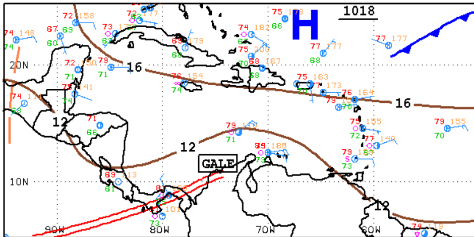
Figura 1: Situación meteorológica actual en el Mar Caribe y Océano Atlántico, enero 23 de 2021, Fuente: NHC NOAA.
