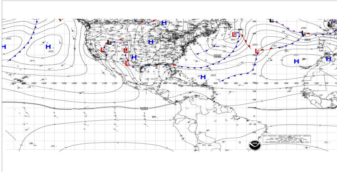
Figura 1: Situación meteorológica actual en el Mar Caribe y Océano Atlántico, enero 23 de 2021, Fuente: NHC NOAA.
