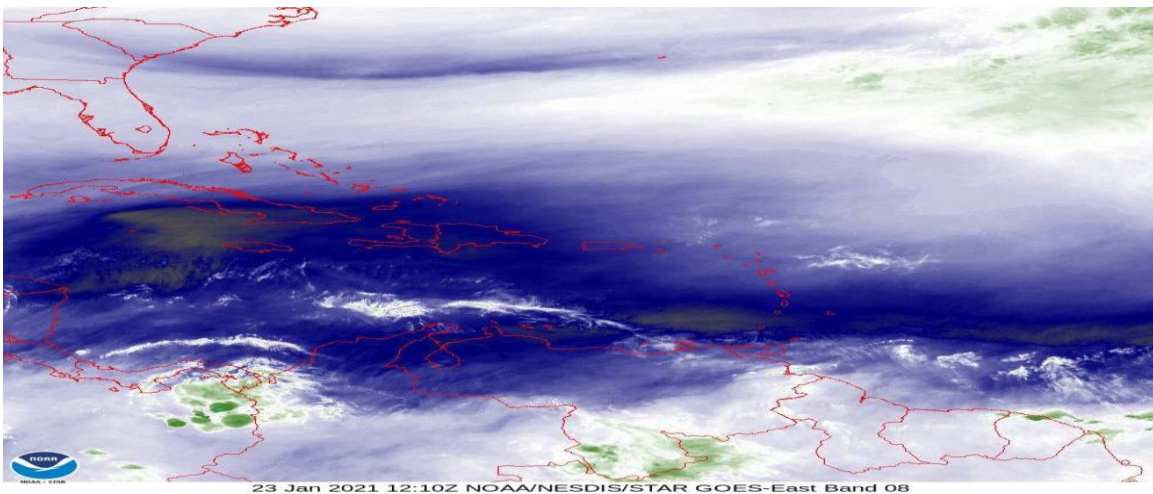
Figura 5: Imagen satelital GOES vapor de agua, enero 23 de 2021, hora 7:00 am de Colombia. Fuente: NOAA.
