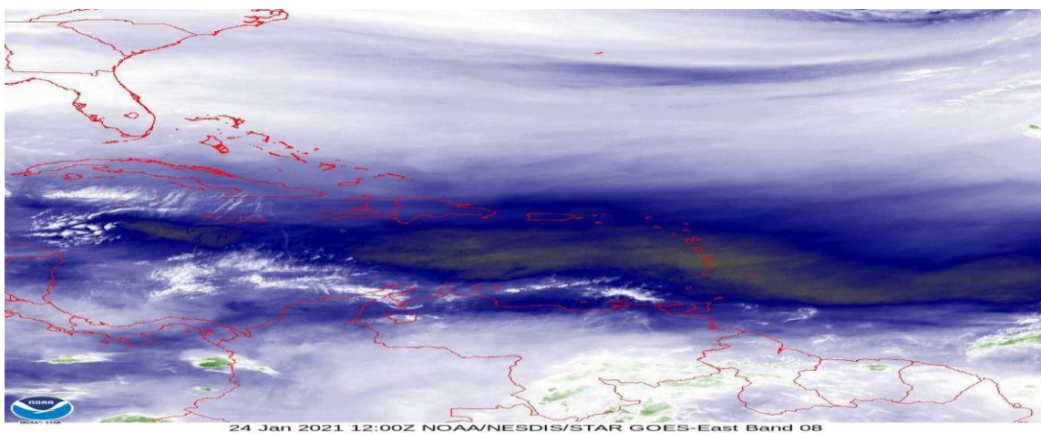
Figura 5: Imagen satelital GOES vapor de agua, enero 24 de 2021, hora 7:00 am de Colombia. Fuente: NOAA.
