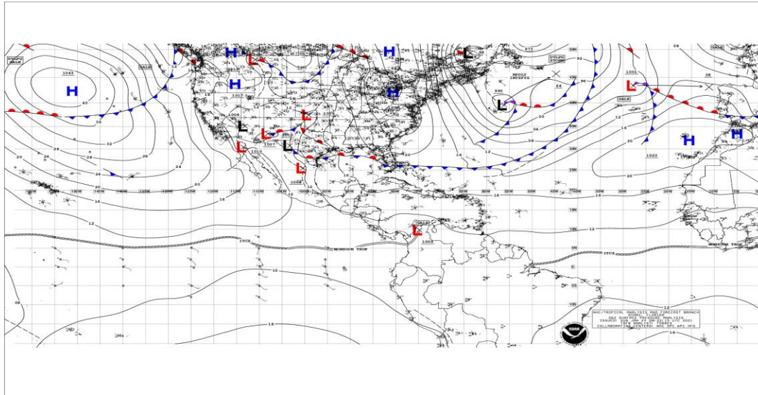
Figura 1: Situación meteorológica actual en el Mar Caribe y Océano Atlántico, enero 24 de 2021, Fuente: NHC NOAA.
