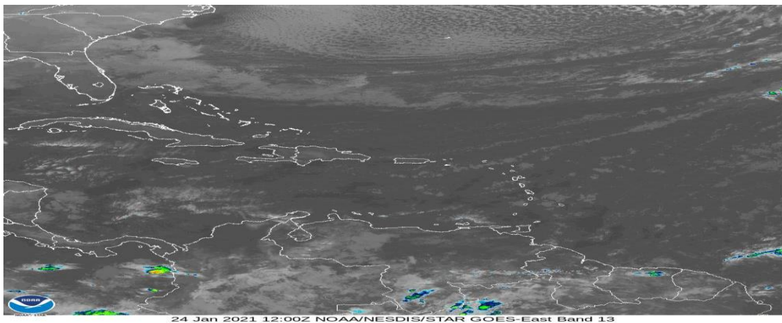
Figura 4: Imagen satelital GOES, enero 24 de 2021, hora 7:00 am de Colombia. Fuente: NOAA.
