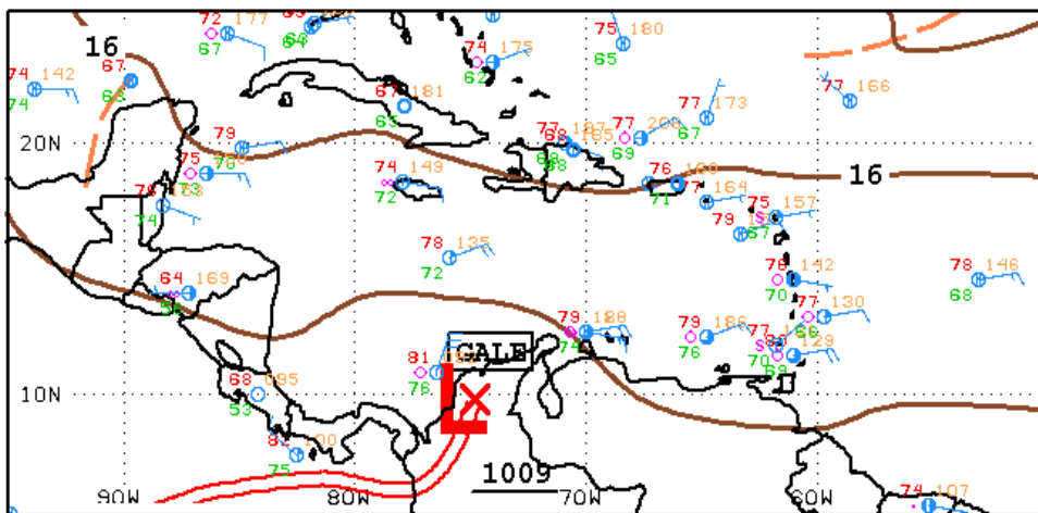
Figura 1: Situación meteorológica actual en el Mar Caribe y Océano Atlántico, enero 24 de 2021, Fuente: NHC NOAA.
