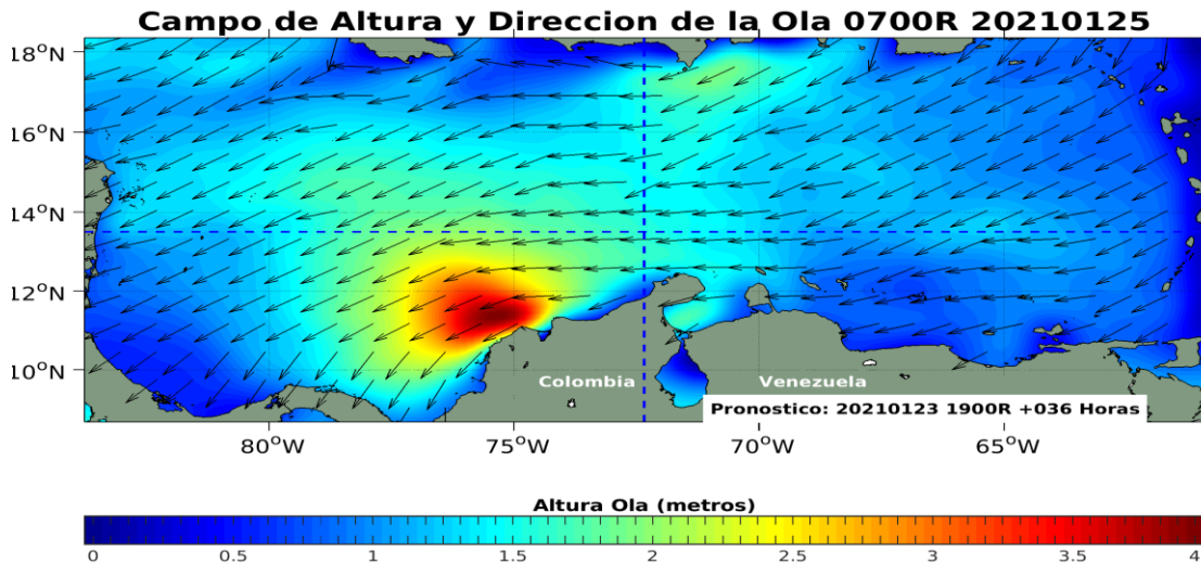
Figura 6: Pronóstico de la altura y dirección de las olas en el Mar Caribe, enero 24 de 2021. Fuente: CIOH.
